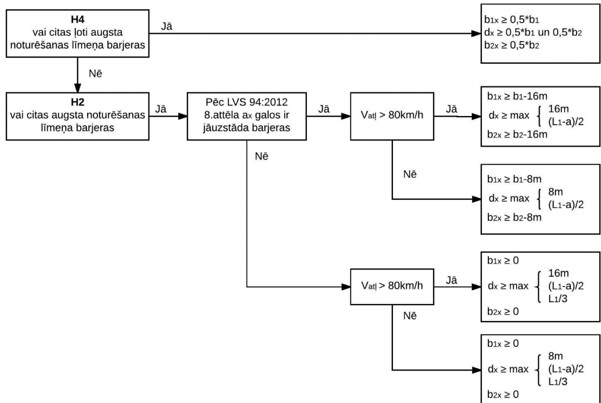
2-24.att. Būvju barjeru aktīvās daļas b_{1x} , b_{2x} un d_x posmu garumu noteikšanas blokshēma.
