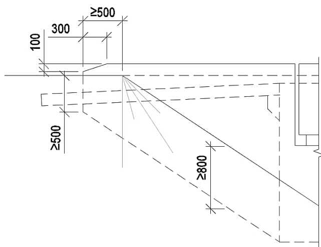
3-10.att. Apmāles nošļaupums tilta galos
