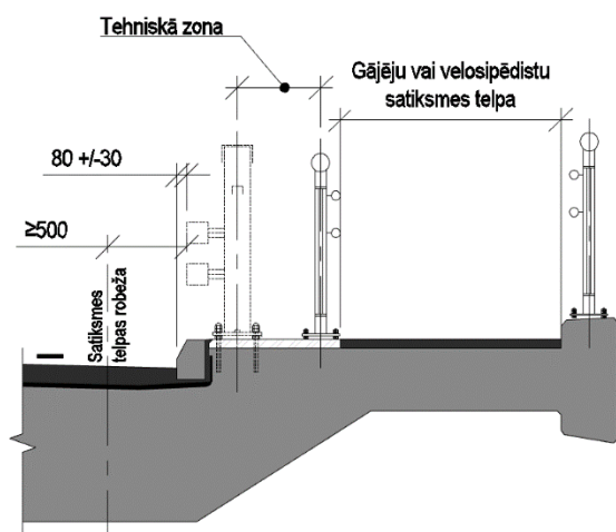
3-5.att. Tilta konstrukcija ar tehnisko zonu
