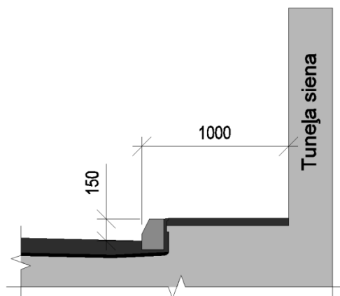
3-7. att. Brauktuves šķērsprofila elementi tunelī bez gājēju ietves.
