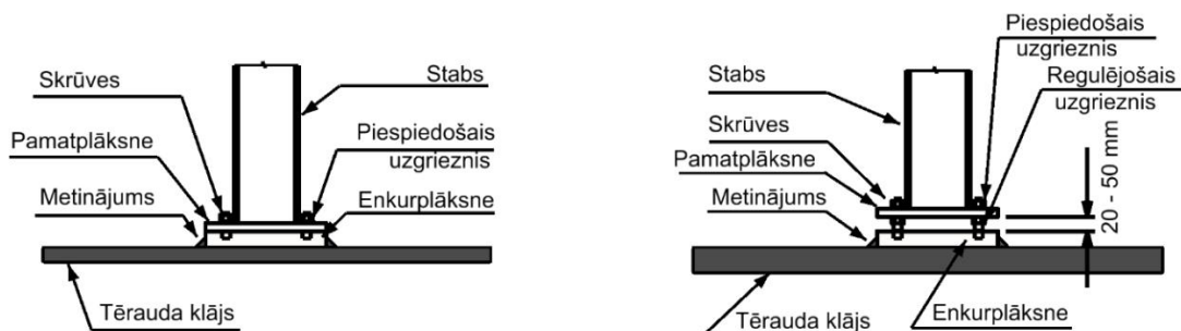
3-12.att. Piemērs margu vai barjeru staba stiprinājumam pie tērauda klāja.
