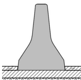
2-5.att. Seguma dilumkārtā nostiprināta barjera
