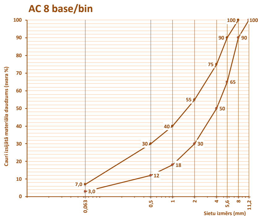
6.2-34 tabula. Prasības karstā asfalta AC 8 base/bin granulometriskajam sastāvam
