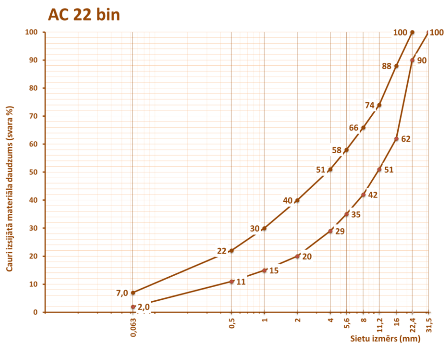
6.2-46 tabula. Prasības karstā asfalta AC 22 bin granulometriskajam sastāvam
