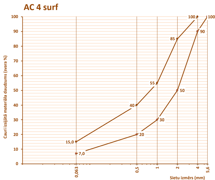
6.2-16 tabula. Prasības karstā asfalta AC 4 surf granulometriskajam sastāvam
