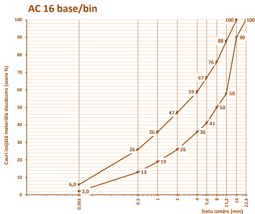
6.2-40 tabula. Prasības karstā asfalta AC 16 base/bin granulometriskajam sastāvam
