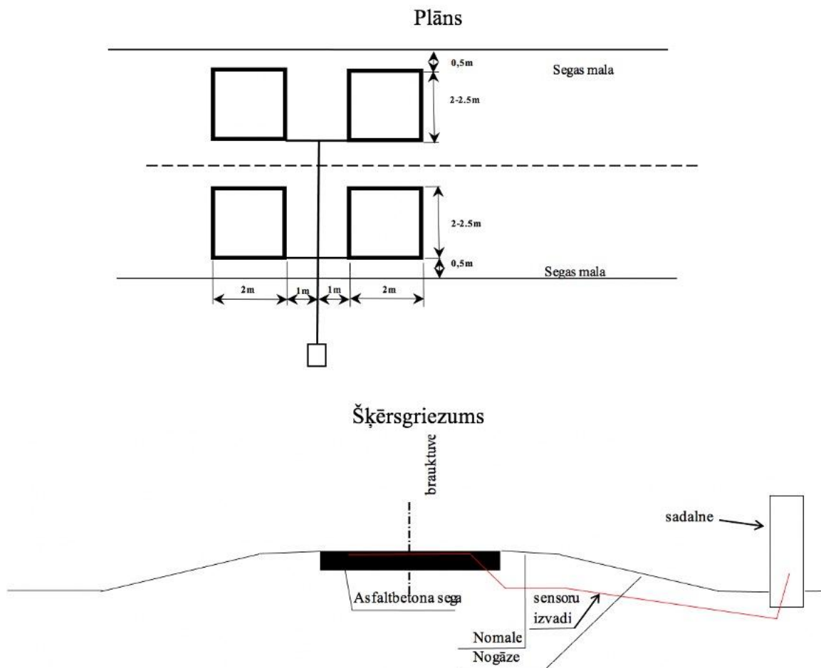
7.13-2 attēls. Satiksmes intensitātes uzskaites punkta izbūves novietojums.
