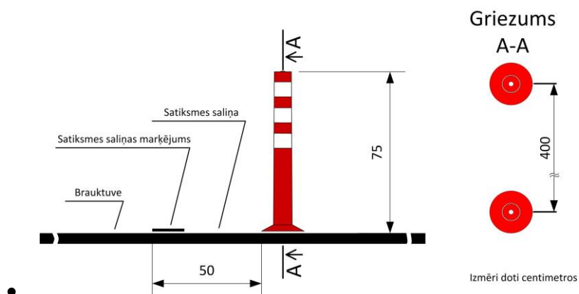
7.5-2 attēls. "Signālstabiņa uzstādīšana".
