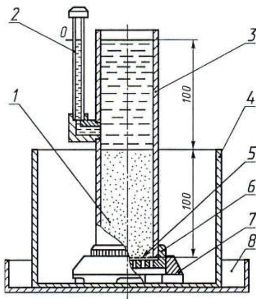
9.3-1 attēls. Smilšainu grunts filtrācijas koeficienta noteikšanas aparāts
