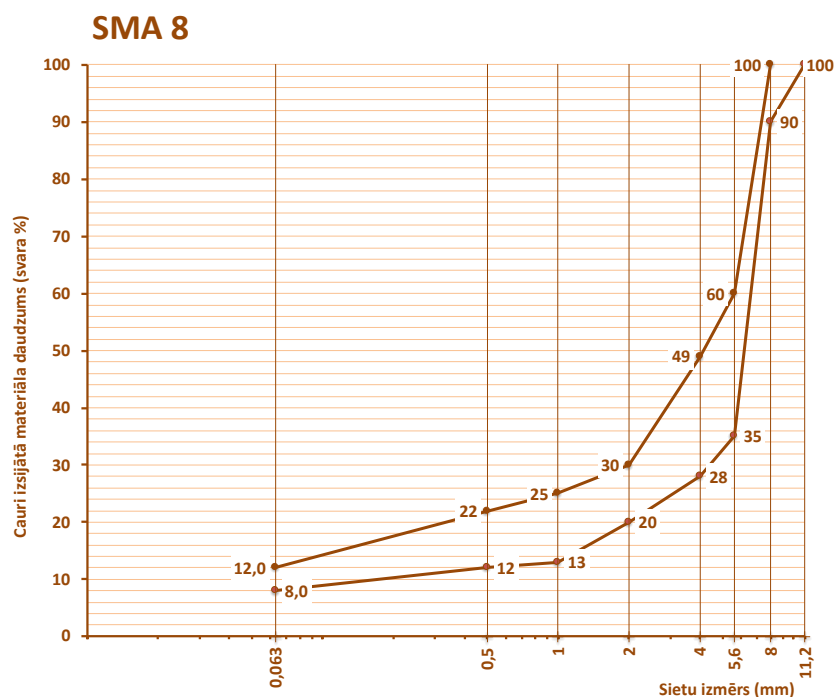
6.2-50 tabula. Prasības šķembu mastikas asfalta SMA 8 granulometriskajam sastāvam
