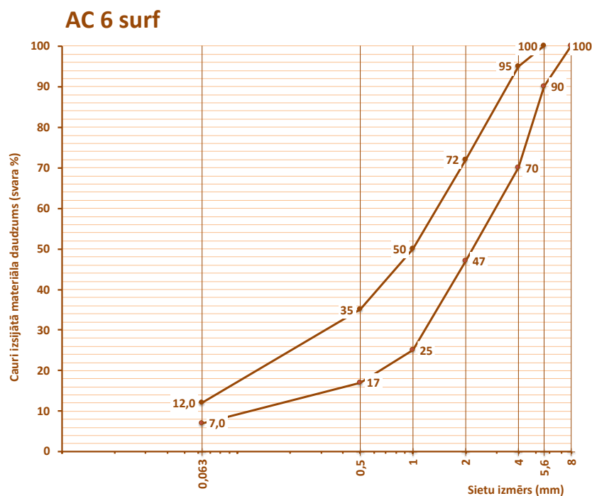
6.2-19 tabula. Prasības karstā asfalta AC 6 surf granulometriskajam sastāvam
