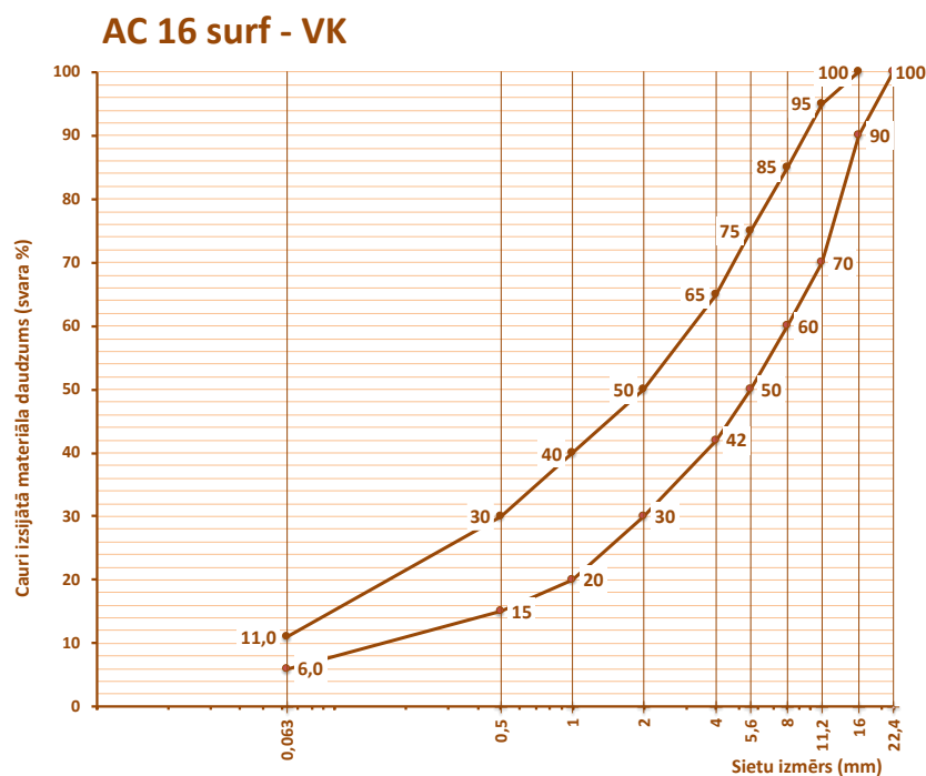
6.2-31 tabula. Prasības karstā asfalta AC 16 surf – VK granulometriskajam sastāvam
