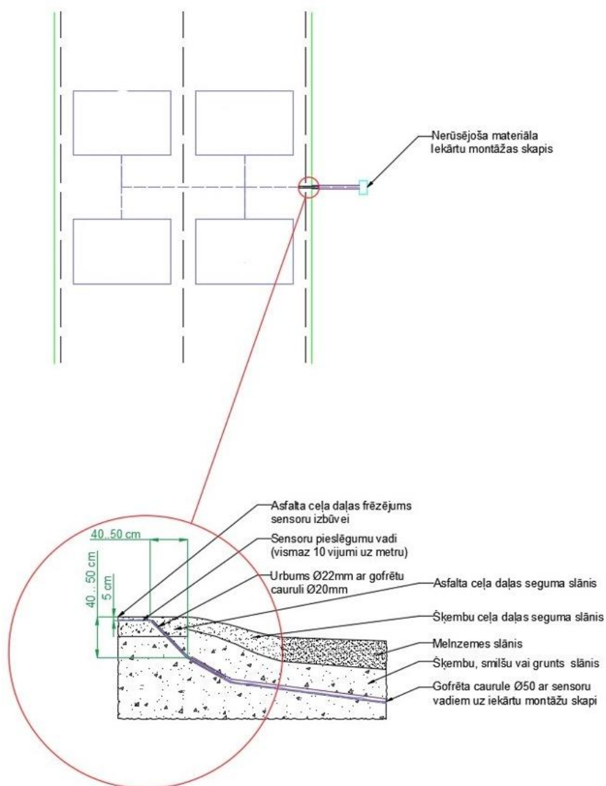
7.13-1 attēls. Sensoru izvietojums un pāreja asfalts/zemes klātne. Sensoru izvietojums: 1. un 2. joslā ar pieaugošu piketāžu, 3. un 4. joslā ar dilstošu piketāžu, pirmajam šķērsojamam sensoram jābūt ar mēzāko skaitli.
