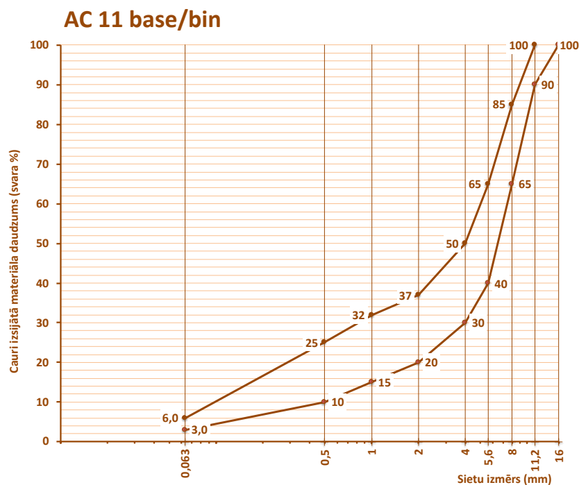
6.2-37 tabula. Prasības karstā asfalta AC 11 base/bin granulometriskajam sastāvam
