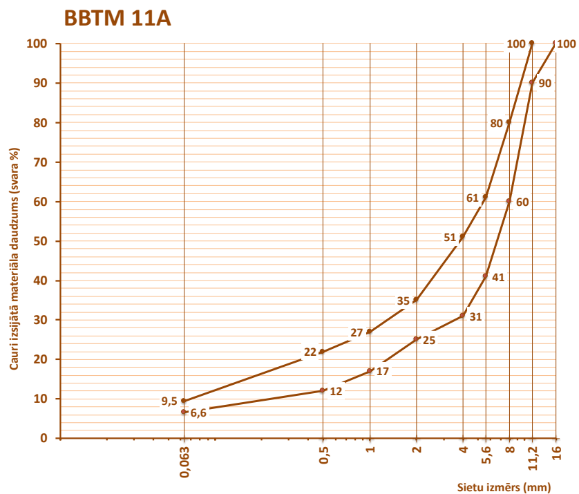
6.5-10 tabula. BBTM 11A granulometriskais sastāvs atbilstoši LVS EN 13108-2
