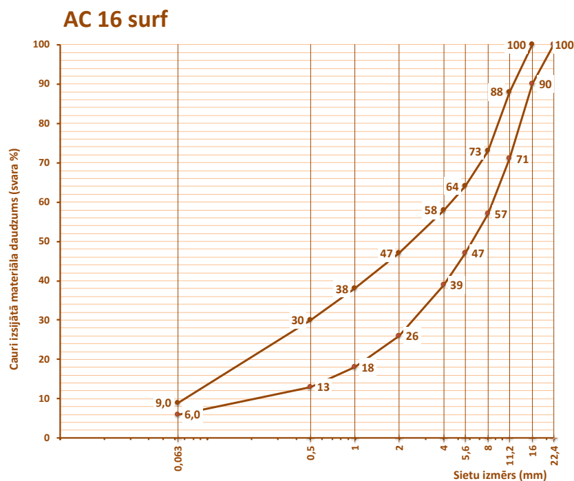
6.2-28 tabula. Prasības karstā asfalta AC 16 surf granulometriskajam sastāvam
