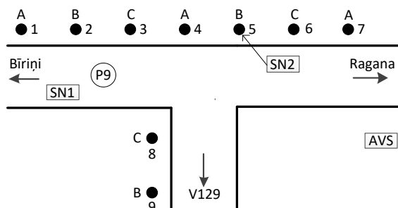
7.12-1 attēls. Izpildshēmas piemēri
