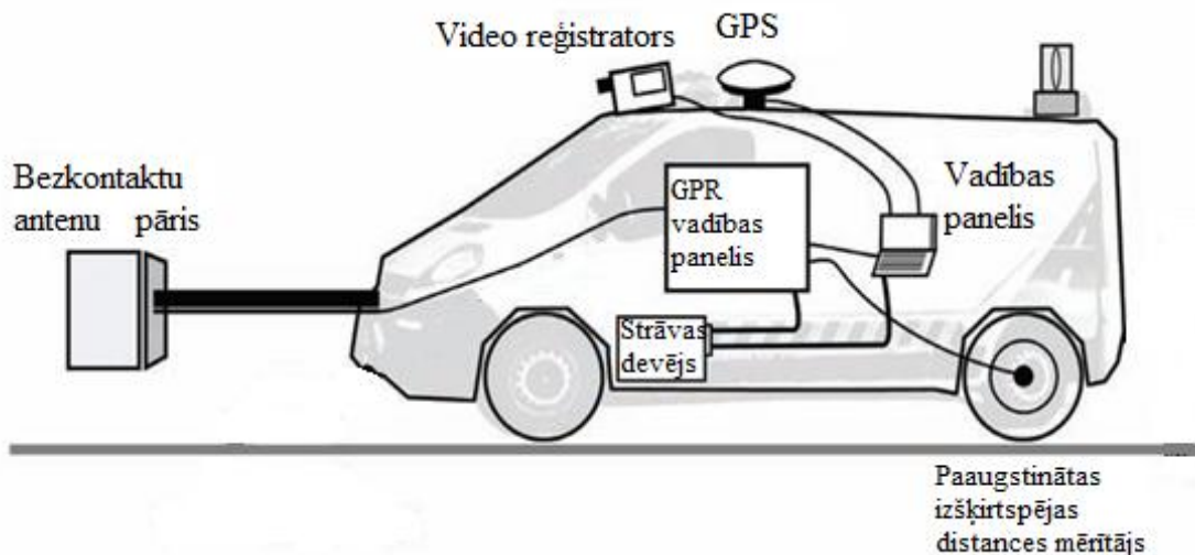
9.12-1 attēls. Mērījumiem izmantotā GPR iekārta
