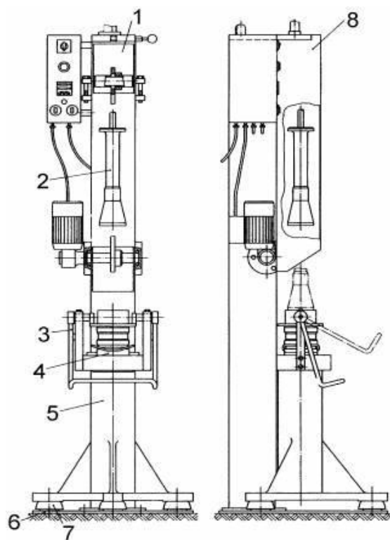
9.8-1 attēls. Trieciena blīvētāja shematisks attēls
