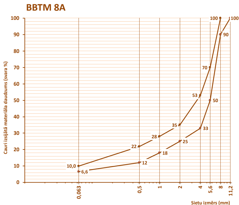
6.5-8 tabula. BBTM 8A granulometriskais sastāvs atbilstoši LVS EN 13108-2
