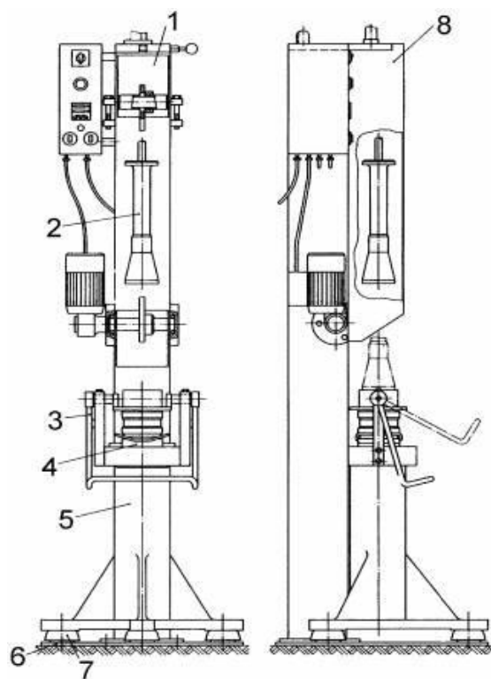
8.8-1 attēls. Trieciena blīvētāja shematiskais attēls
