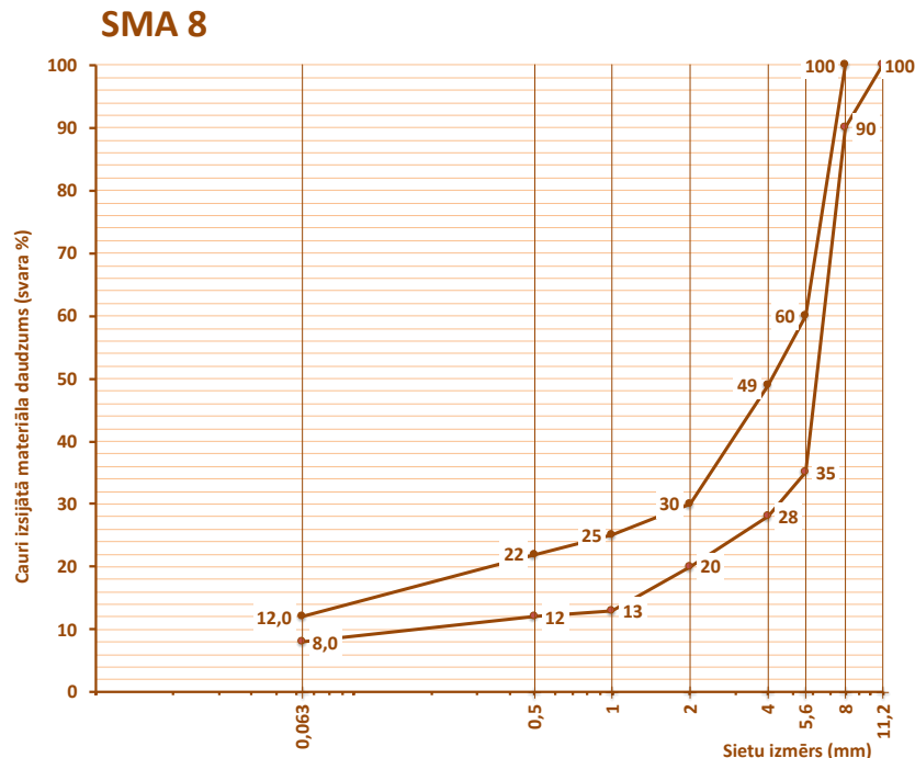
6.2-46 tabula. Prasības šķembu mastikas asfalta SMA 8 granulometriskajam sastāvam
