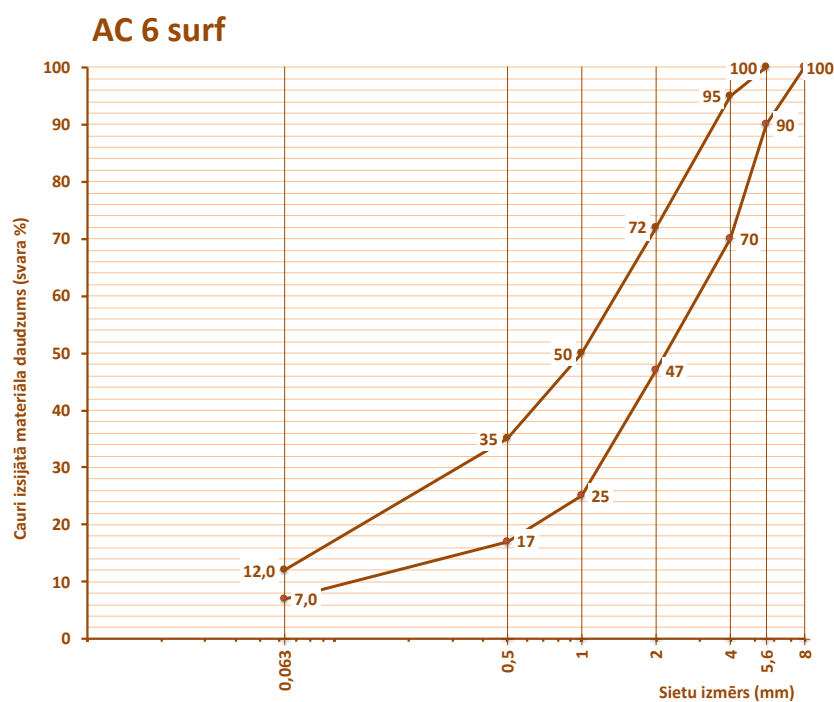
6.2-18 tabula. Prasības karstā asfalta AC 6 surf granulometriskajam sastāvam
