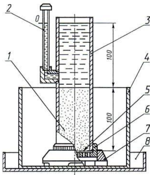
8.3-1 attēls. Smilšainu grunts filtrācijas koeficienta noteikšanas aparāts
