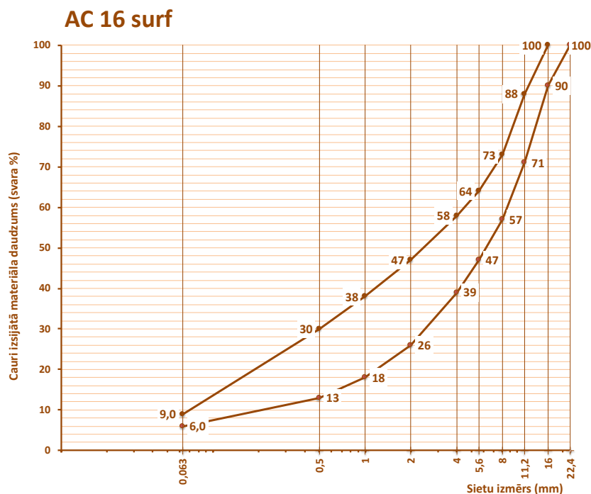
6.2-27 tabula. Prasības karstā asfalta AC 16 surf granulometriskajam sastāvam
