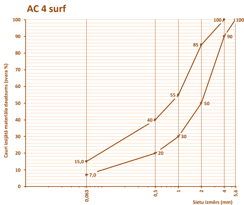
6.2-15 tabula. Prasības karstā asfalta AC 4 surf granulometriskajam sastāvam
