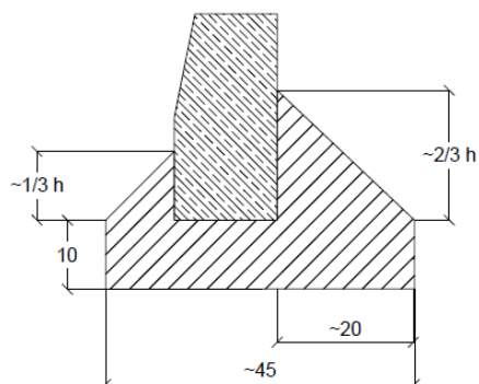
7.2-1 attēls. Apmāļu nostiprinājuma betonā skices
