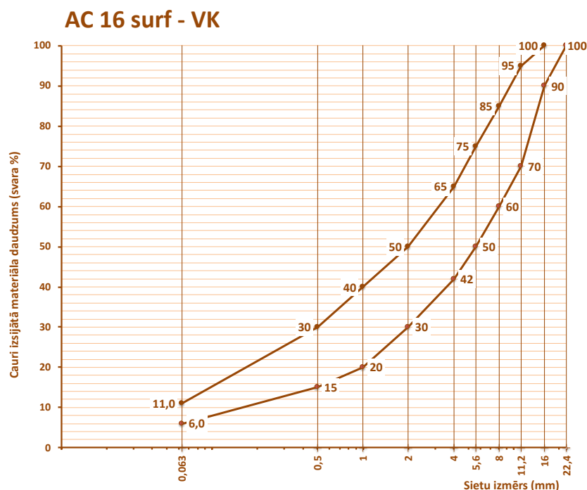
6.2-30 tabula. Prasības karstā asfalta AC 16 surf – VK granulometriskajam sastāvam
