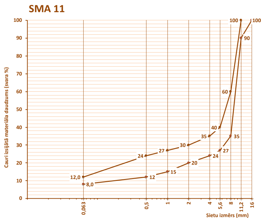
6.2-49 tabula. Prasības šķembu mastikas asfalta SMA 11 granulometriskajam sastāvam
