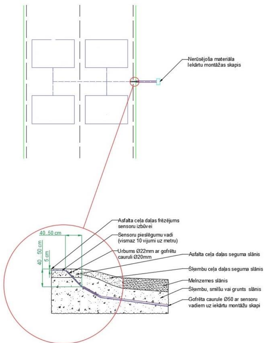
7.12-1 attēls. Sensoru izvietojums un pāreja asfalts/zemes klātne. Sensoru izvietojums: 1. un 2. joslā ar pieaugošu piketāžu, 3. un 4. joslā ar dilstošu piketāžu, pirmajam šķērsojamam sensoram jābūt ar mazāko skaitli.
