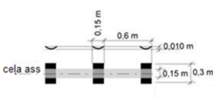
7.13-2 Attēls. Darbu izpildes tehnoloģiskā shēma
