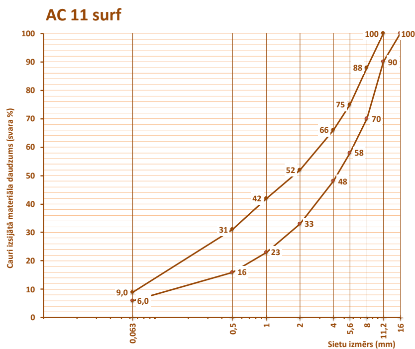
6.2-24 tabula. Prasības karstā asfalta AC 11 surf granulometriskajam sastāvam
