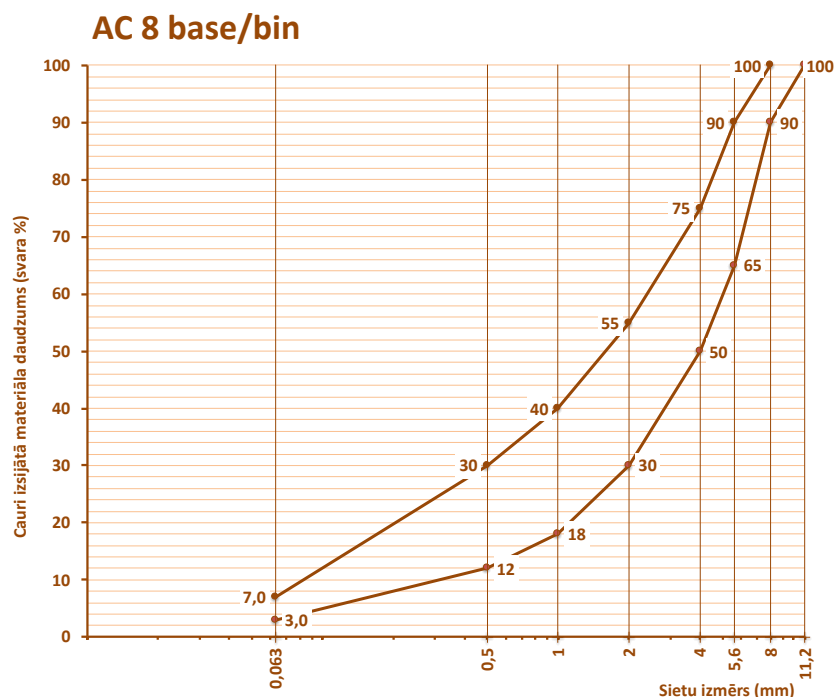
6.2-33 tabula. Prasības karstā asfalta AC 8 base/bin granulometriskajam sastāvam
