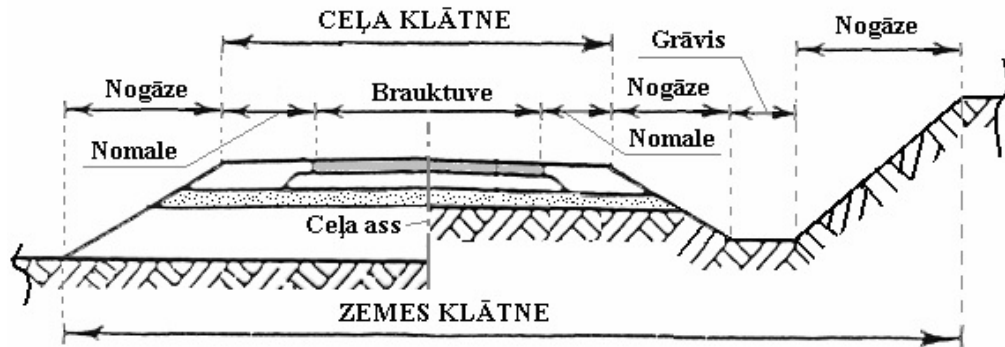
1.1-2 attēls. Ceļa konstrukcija
