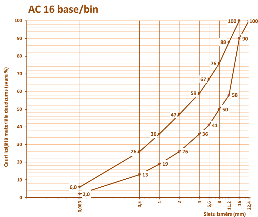
6.2-39 tabula. Prasības karstā asfalta AC 16 base/bin granulometriskajam sastāvam
