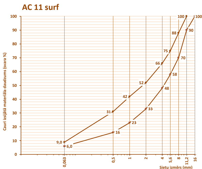
6.2-24 tabula. Prasības karstā asfalta AC 11 surf granulometriskajam sastāvam
