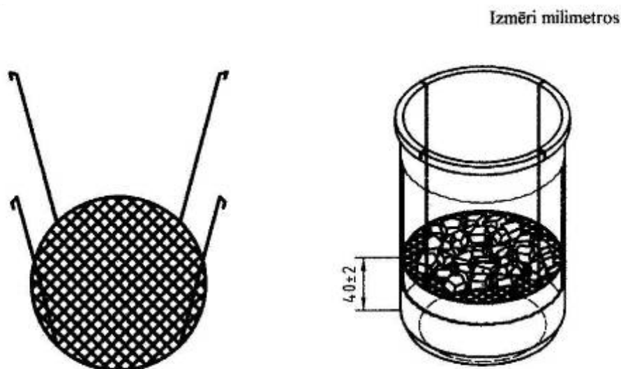
A . attēls. Atbalsta tīkliņš ar āķiem
