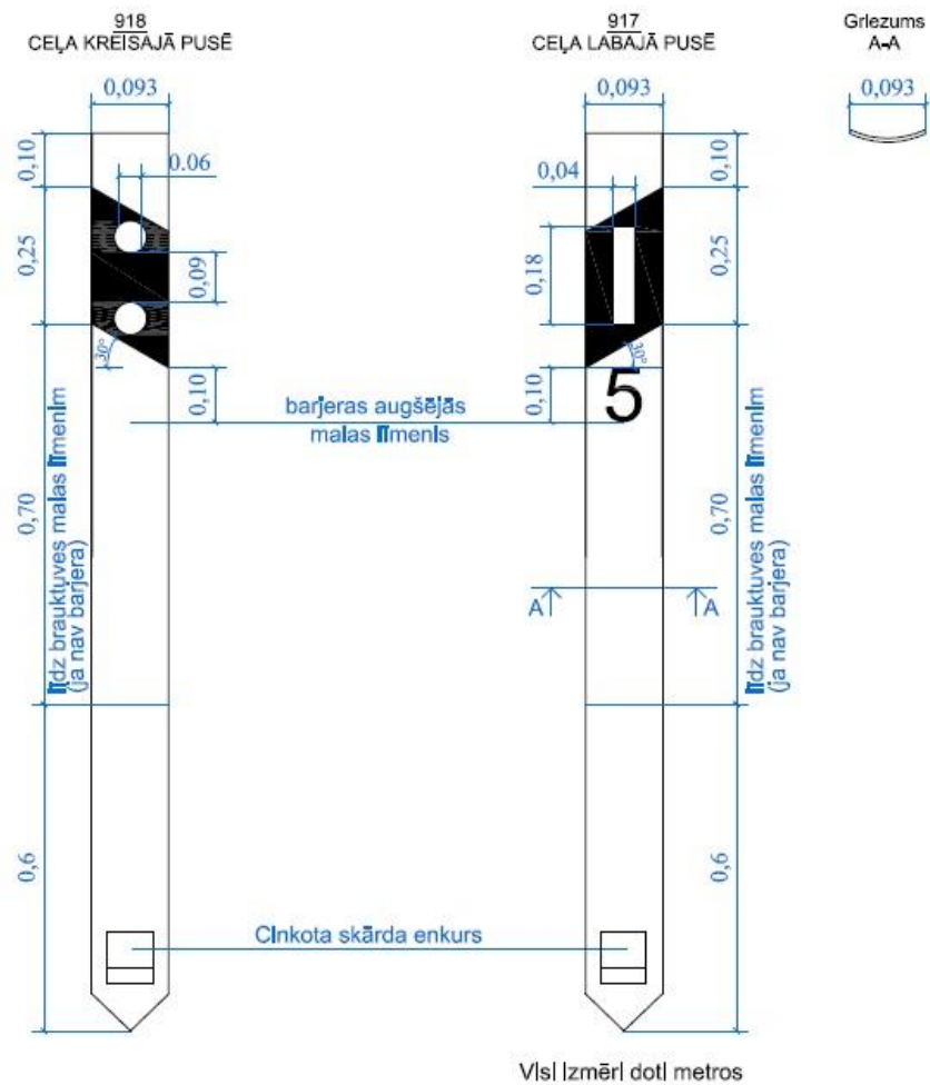
7.4-1 attēls. Signālstabiņi
