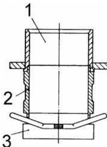
12.8-2 attēls. Triecienu blīvētāja tipiska blīvēšanas veidne
