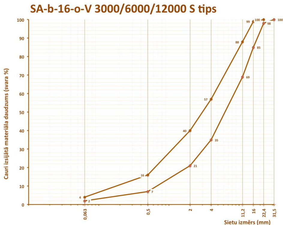
6.3-21 tabula. Prasības mīkstā asfalta SA-b-16-o-V 3000/6000/12000 S tips maisījuma granulometriskajam sastāvam
