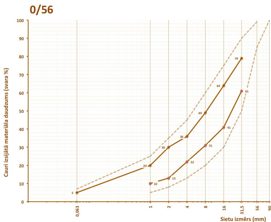
5.2-19 tabula. Prasības 0/56 maisījuma granulometriskajam sastāvam
