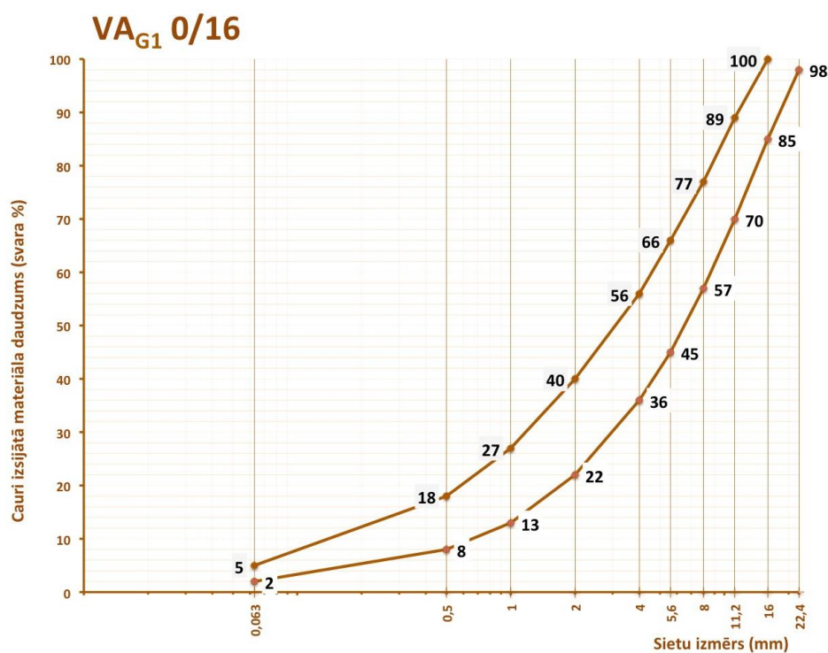
6.6-8 tabula. Prasības VA G1 0/16 granulometriskajam sastāvam
