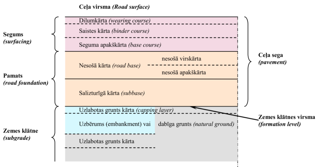
1.1-1 attēls. Ceļa konstruktīvās kārtas
