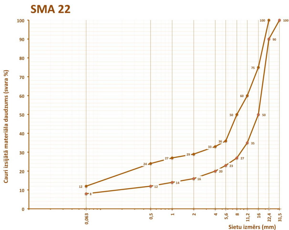
6.2-65 tabula. Prasības šķembu mastikas asfalta SMA 22 granulometriskajam sastāvam
