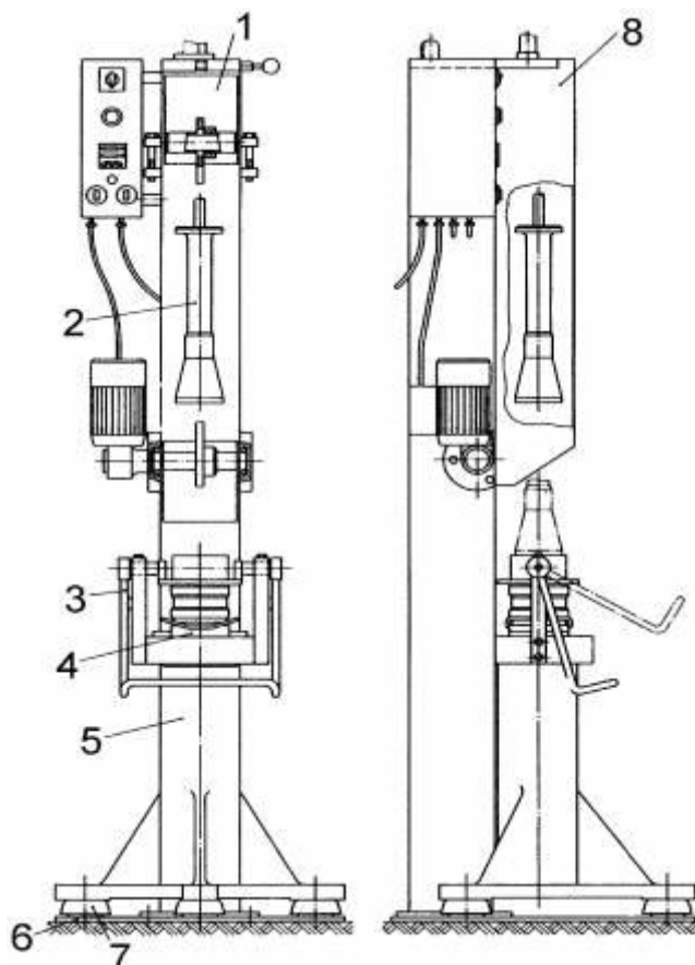
1. attēls. Trieciena blīvētāja shematiskais attēls
