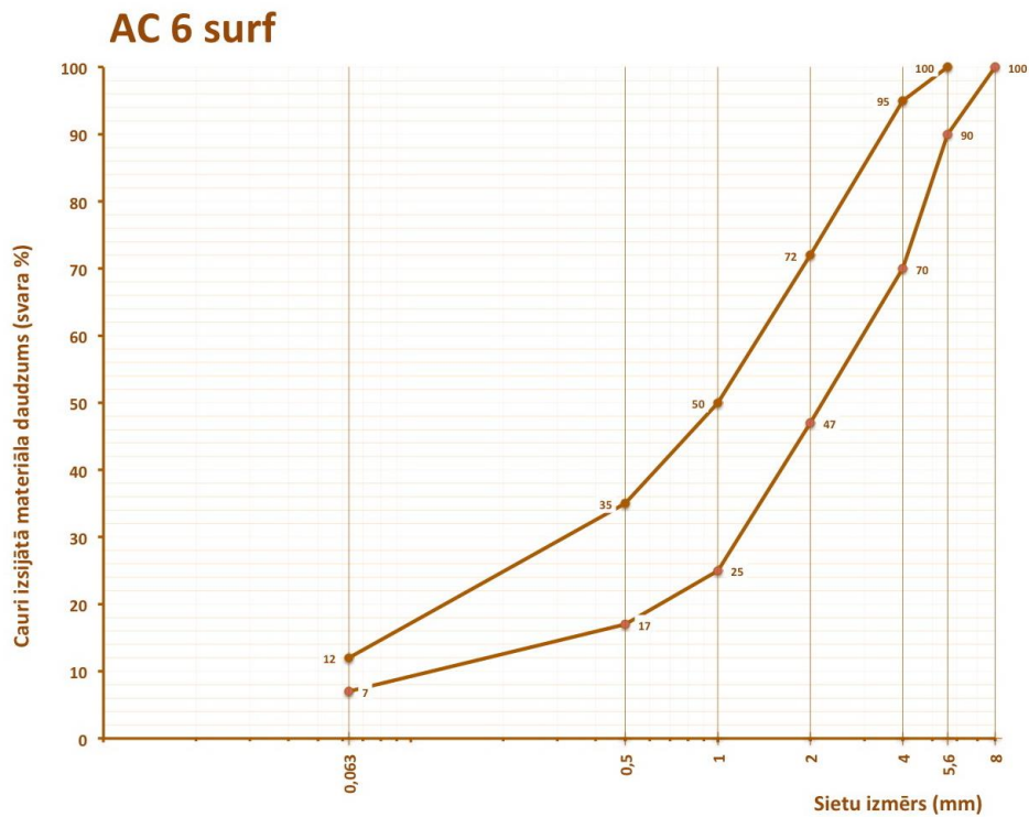
6.2-18 tabula. Prasības karstā asfalta AC 6 surf granulometriskajam sastāvam
