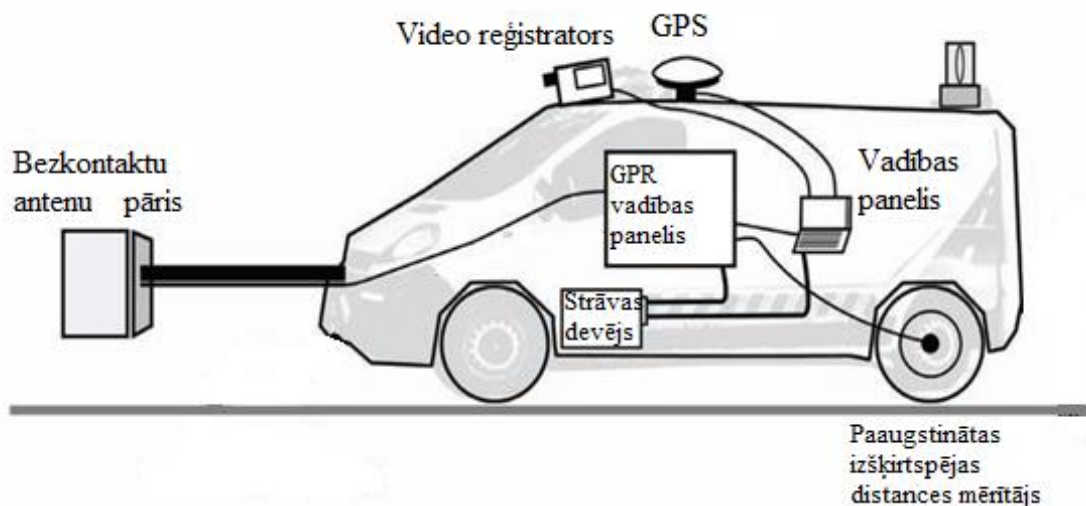
8.13-1 attēls. Mērījumiem izmantotā GPR iekārta
