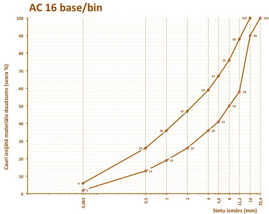
6.2-39 tabula. Prasības karstā asfalta AC 16 base/bin granulometriskajam sastāvam
