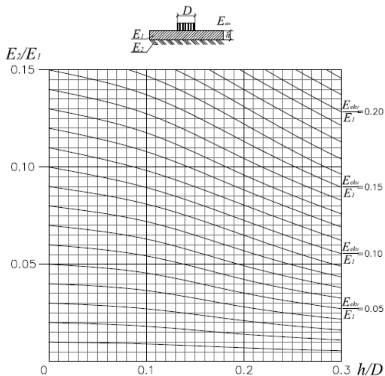
Att. P9.1. Nomogrammas (sk. att. P9.2) detaļa koeficienta E_{ekv}/E_2 noteikšanai bituminētajās kārtās.
