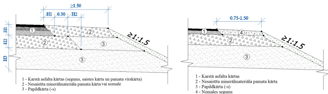
2.1. att. Ja nomaļes platums ir >1.50
