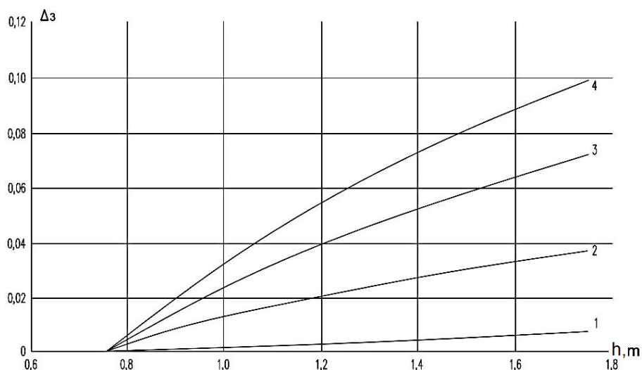
Att. P.2.1. Grafiks segas stabilo kārtu biezuma korekcijas \Delta_3 noteikšanai
