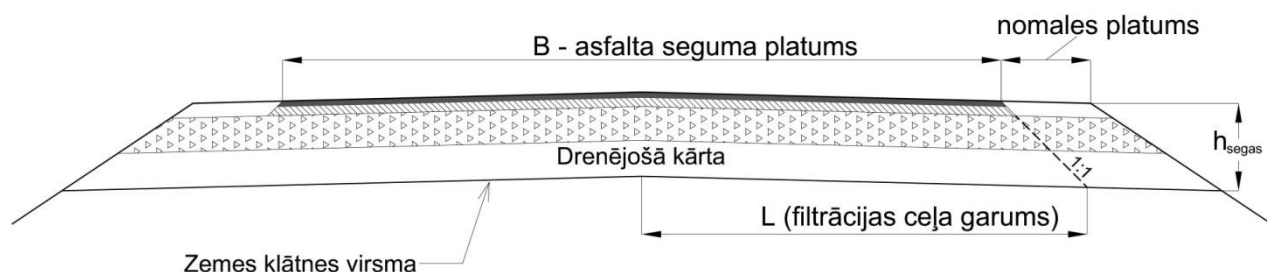
Att. 5.2. Filtrācijas ceļa (L) noteikšana
