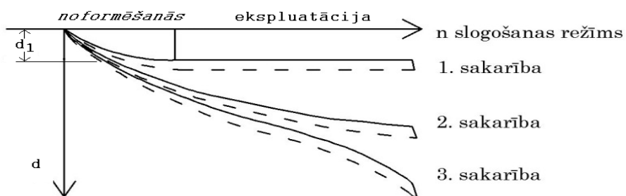
3. att. Segas darbība atkarībā no sloģšanas režīma un grunts nestspējas
