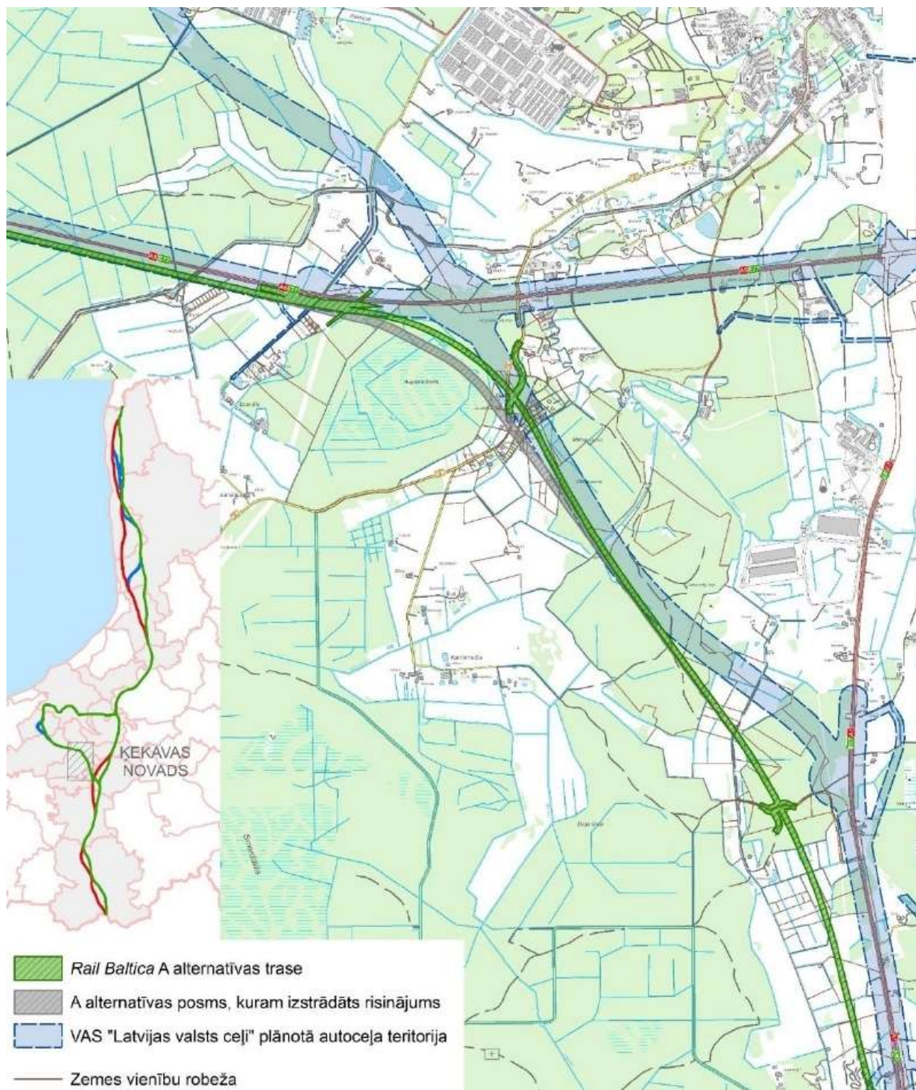
2.4.13. attēls. Rail Baltica trase Ķekavas apvedceļa zonā
