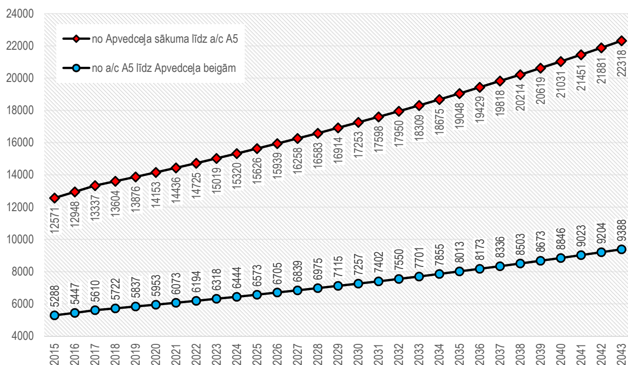
2.1.1. attēls. Intensitātes prognoze Ķekavas apvedceļam
