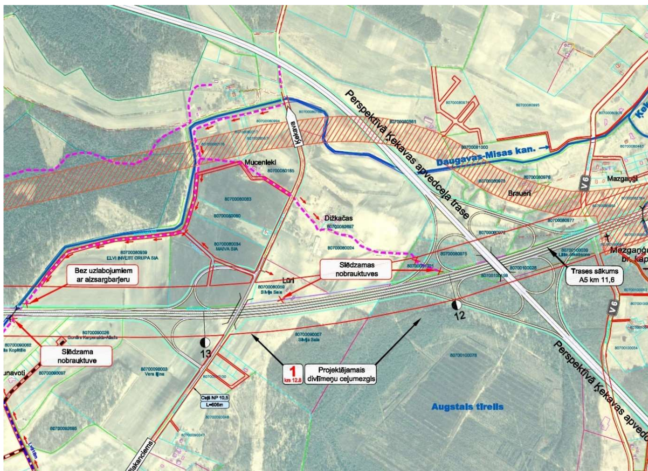
2.4.11.attēls. Autoceļa A5 rekonstrukcija Ķekavas apvedceļa zonā
