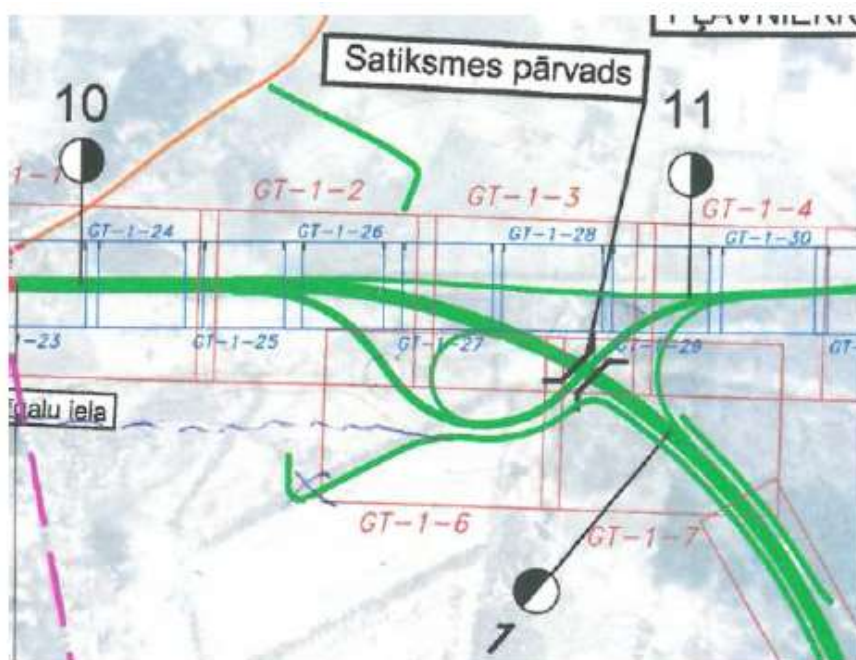
0.2. attēls. Ķekavas apvedceļa sākuma mezgls a/c A7 10,3 km, 2008.gads.
