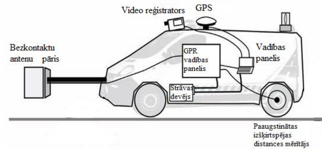
12.13-1 attēls. Mērījumiem izmantotā GPR iekārta
