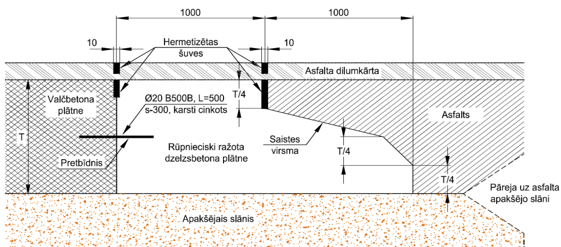
6.4-66.5-6 attēls. Salaiduma šuve ar pārejas plātņi
