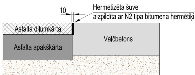
6.4-46.5-4 attēls. Standarta salaiduma šuve
