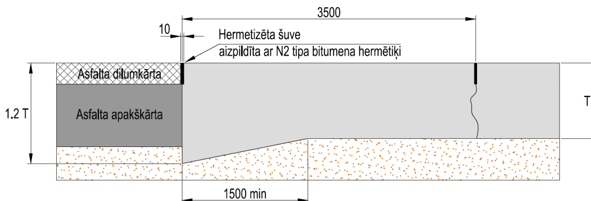
6.4-56.5-5 attēls. Salaiduma šuve ar sabiezinātu betona malu
