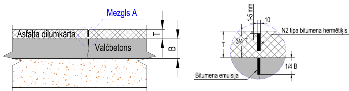
6.4-36.5-3 attēls. Šuves konstrukcija asfalta dilumkārtā
