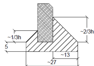
Betona apmale 100x20x8 cm
