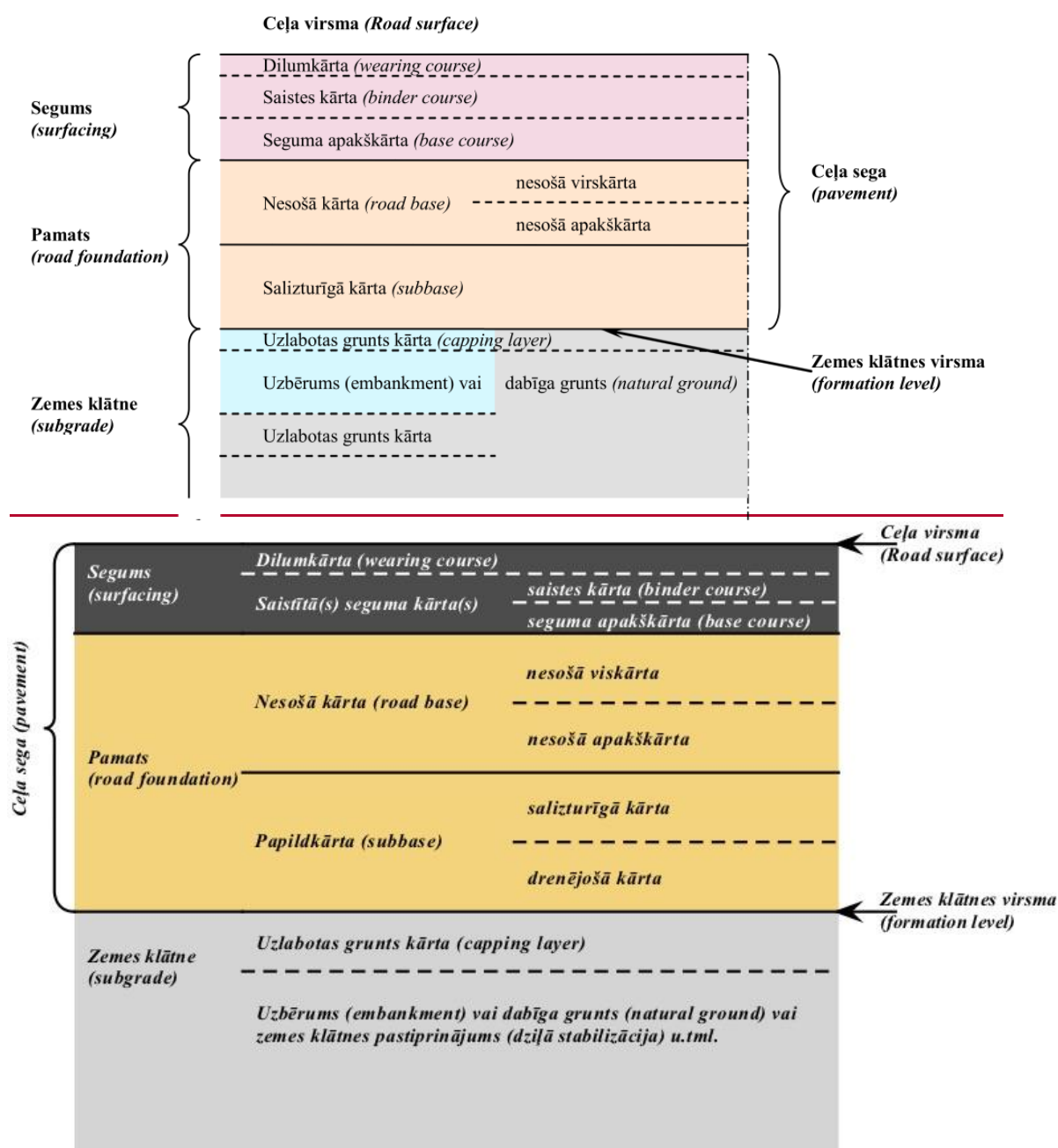
1.1-1 attēls. Ceļa konstruktīvās kārtas
