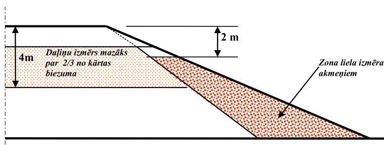
4.4-1 attēls. Zemes klātnes uzbēruma zonas
