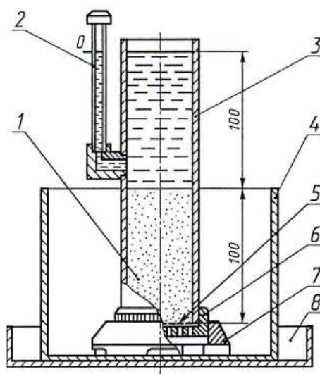
12.3-1 attēls. Smilšainu grunts filtrācijas koeficienta noteikšanas aparāts
