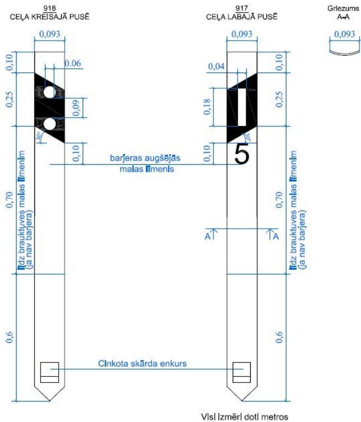
7.4-1 attēls. Signālstabiņi
