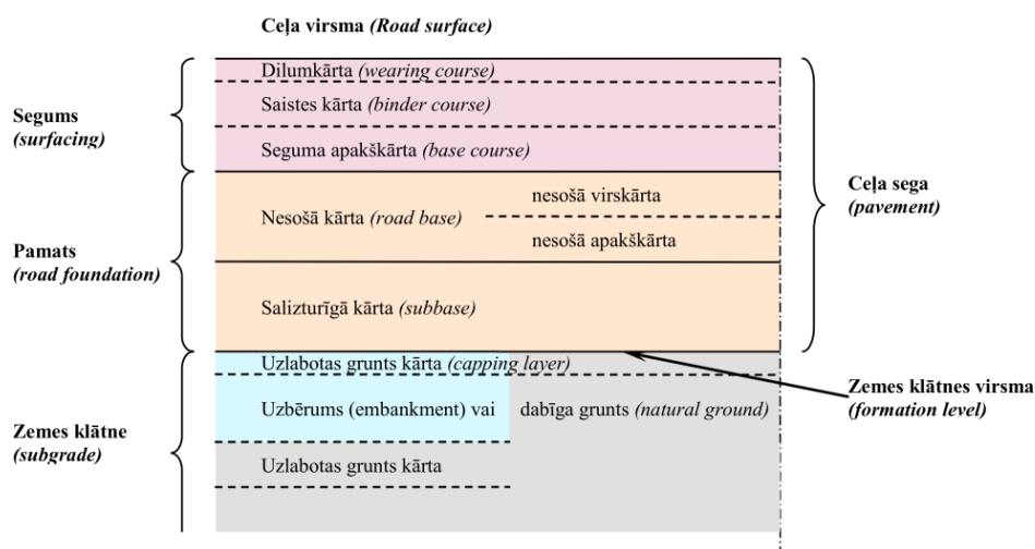
1.1-1 attēls. Ceļa konstruktīvās kārtas
