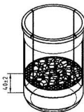
B.attēls. Testēšanas paraugs ievietots vārglāzē
