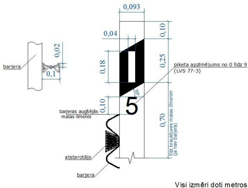
7.4-2 attēls. Signālstabiņi virs barjeras
