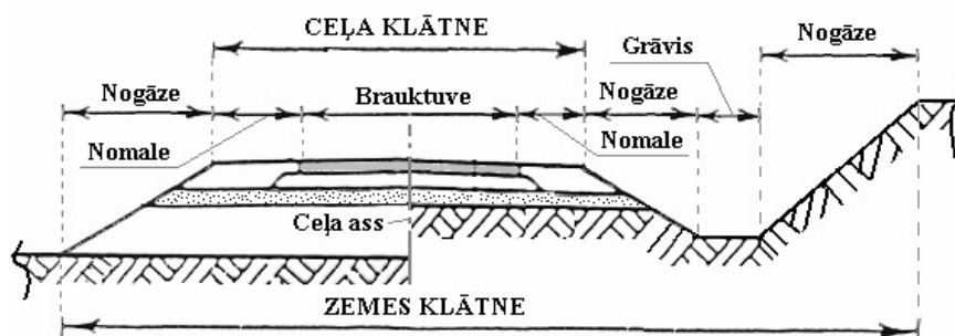
1.1-2 attēls. Ceļa konstrukcija
