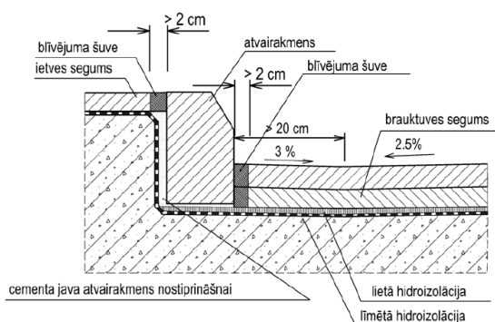
9.24-1 attēls. Blīvējuma šuve starp apmali un segumu, un starp segumu un deformācijas šuvi.
