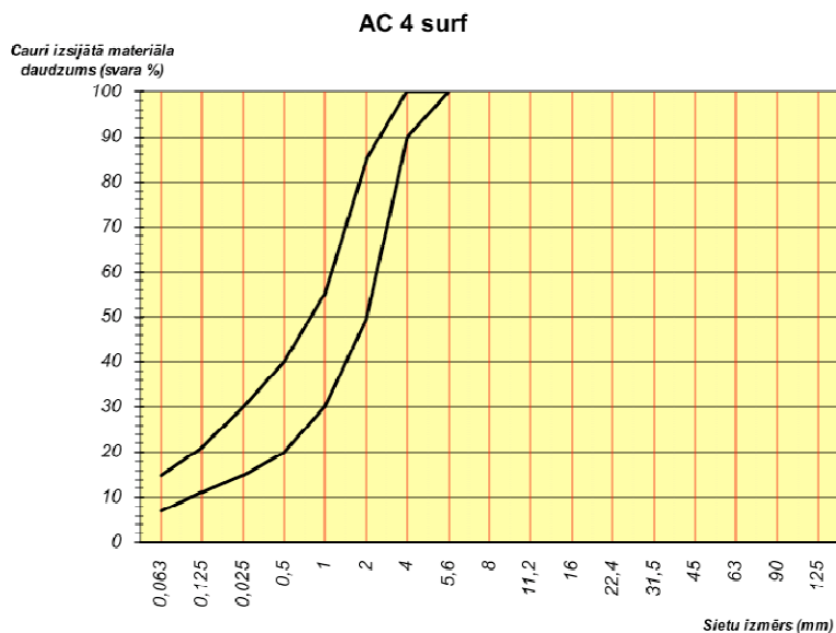
61. tabula. Prasības karstā asfalta AC 4 surf granulometriskajam sastāvam
