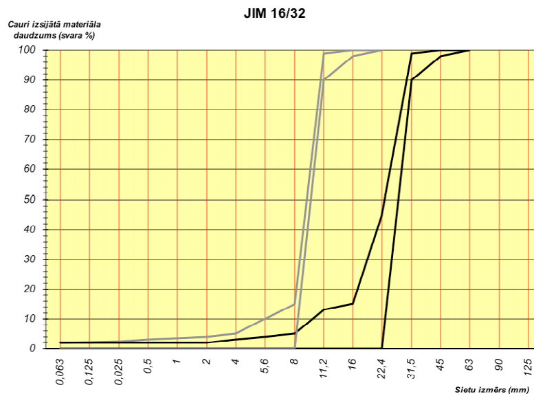
150. tabula. Prasības JIM 16/32 šķembu granulometriskajam sastāvam
