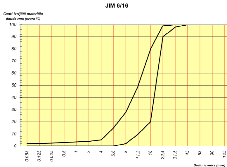
147. tabula. Prasības JIM 6/16 šķembu granulometriskajam sastāvam
