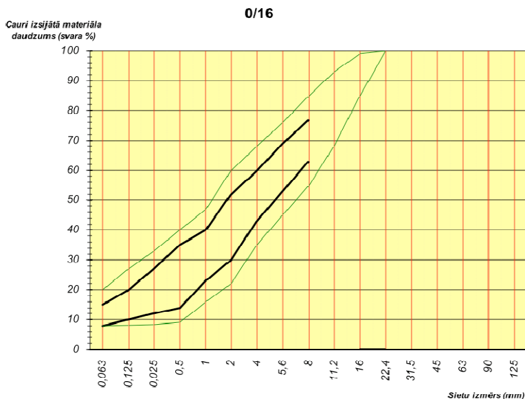
39. tabula. Prasības 0/16 maisījuma granulometriskajam sastāvam
