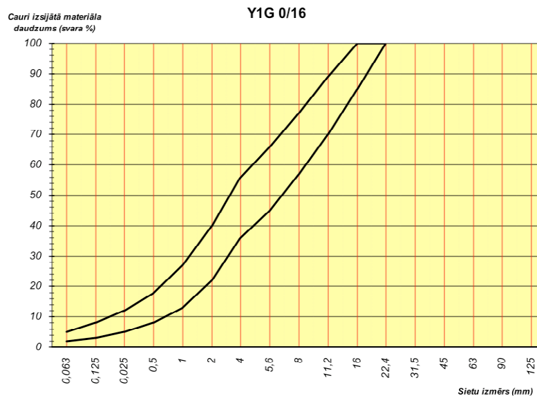
144. tabula. Prasības Y1G 0/16 granulometriskajam sastāvam
