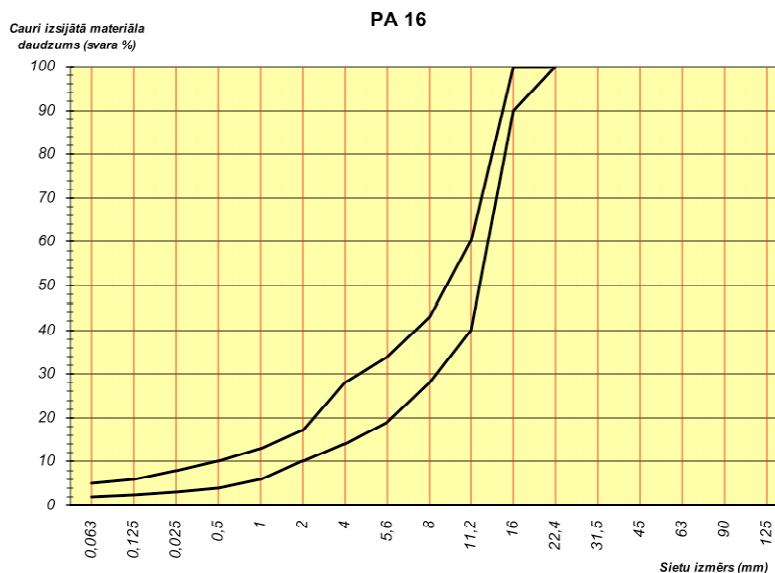
99. tabula. Prasības porasfalta PA 16 granulometriskajam sastāvam
