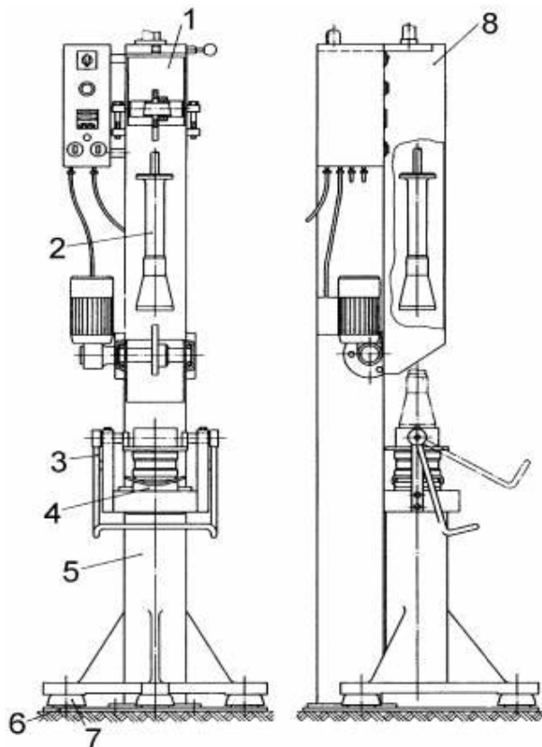
1. attēls. Trieciena blīvētāja shematisks attēls
