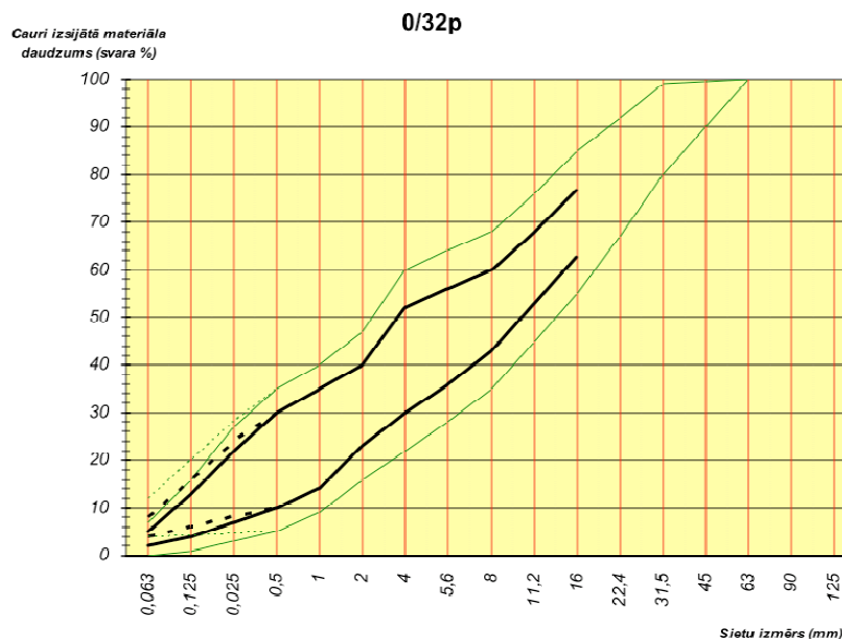
29. tabula. Prasības maisījuma 0/32p granulometriskajam sastāvam Kopīgā granulometriskā sastāva diapazona kategorija – G B
