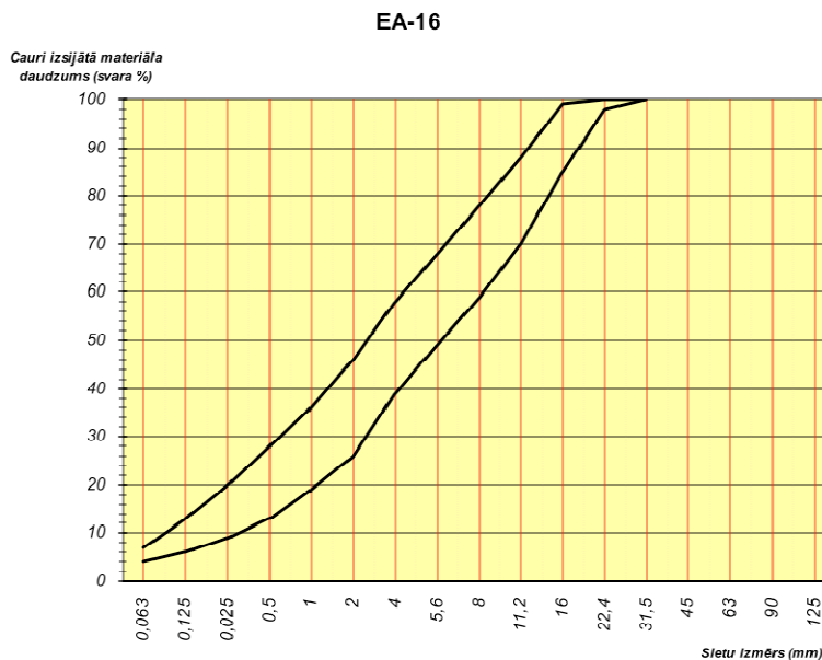
126. tabula. Prasības emulsijas asfalta EA-16 maisījuma granulometriskajam sastāvam
