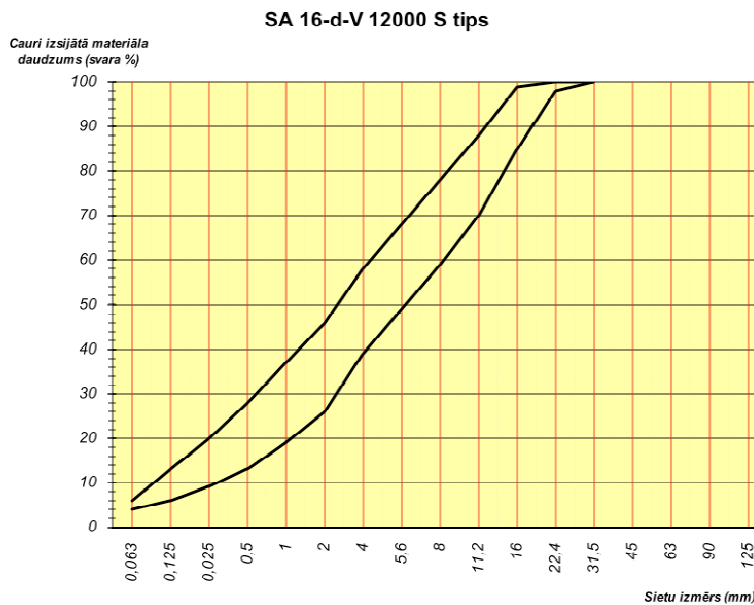
109. tabula. Prasības mīkstā asfalta SA 16-d-V 12000 S tips maisījuma granulometriskajam sastāvam
