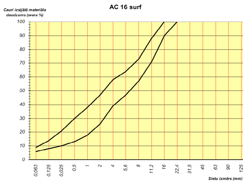
69. tabula. Prasības karstā asfalta AC 16 surf granulometriskajam sastāvam
