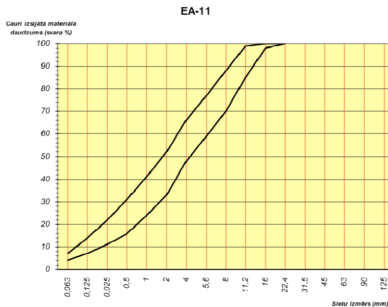
124. tabula. Prasības emulsijas asfalta EA-11 maisījuma granulometriskajam sastāvam
