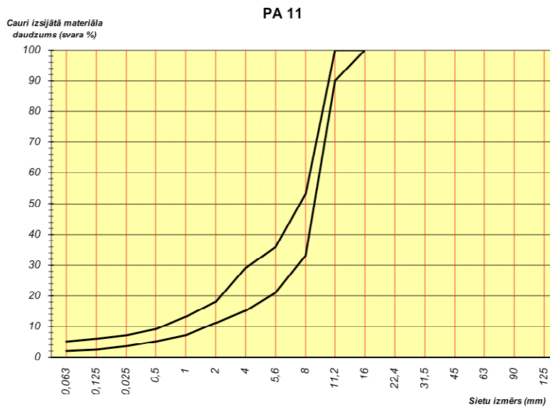
97. tabula. Prasības porasfalta PA 11 granulometriskajam sastāvam
