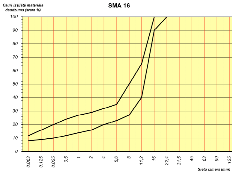
92. tabula. Prasības šķembu mastikas asfalta SMA 16 granulometriskajam sastāvam
