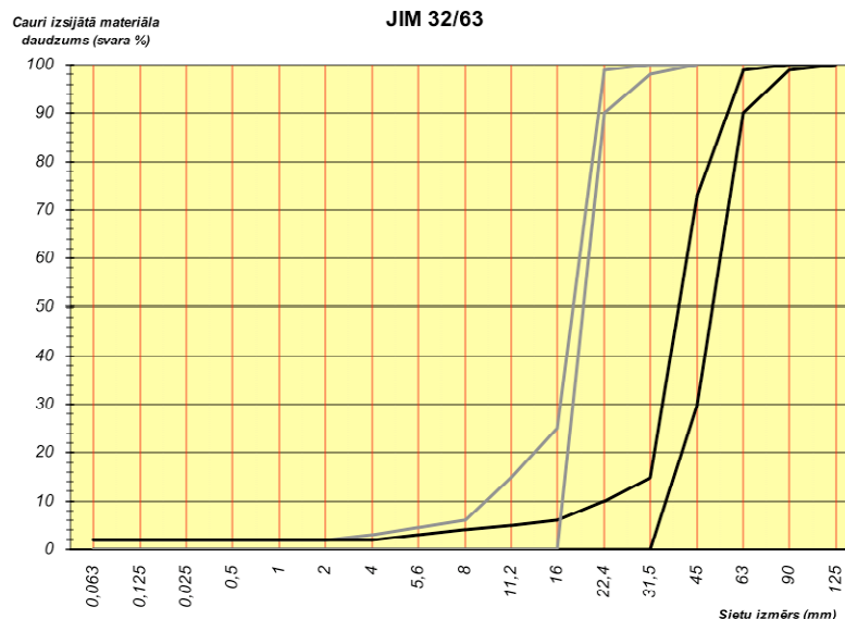
151. tabula. Prasības JIM 32/63 šķembu granulometriskajam sastāvam
