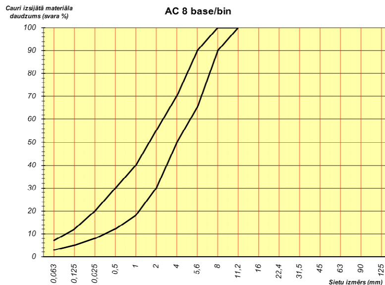
75. tabula. Prasības karstā asfalta AC 8 base/bin granulometriskajam sastāvam
