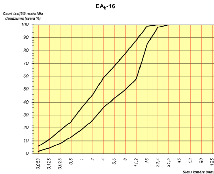
128. tabula. Prasības emulsijas asfalta EA b -16 maisījuma granulometriskajam sastāvam
