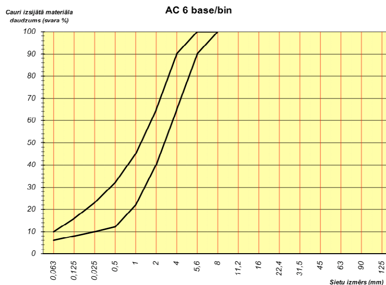
73. tabula. Prasības karstā asfalta AC 6 base/bin granulometriskajam sastāvam
