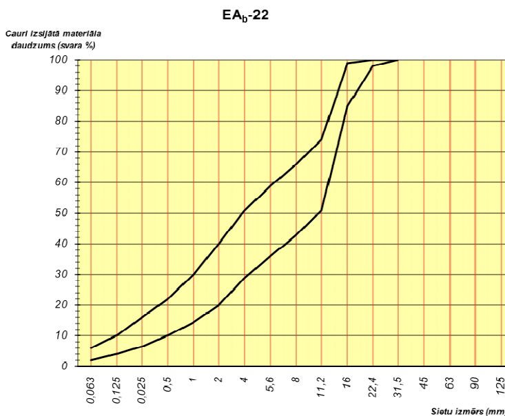
130. tabula. Prasības emulsijas asfalta EA b -22 maisījuma granulometriskajam sastāvam
