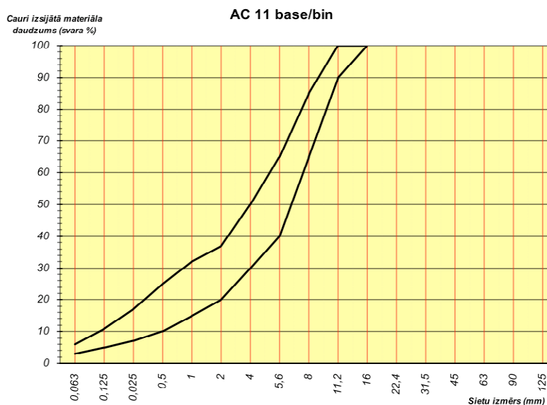
77. tabula. Prasības karstā asfalta AC 11 base/bin granulometriskajam sastāvam
