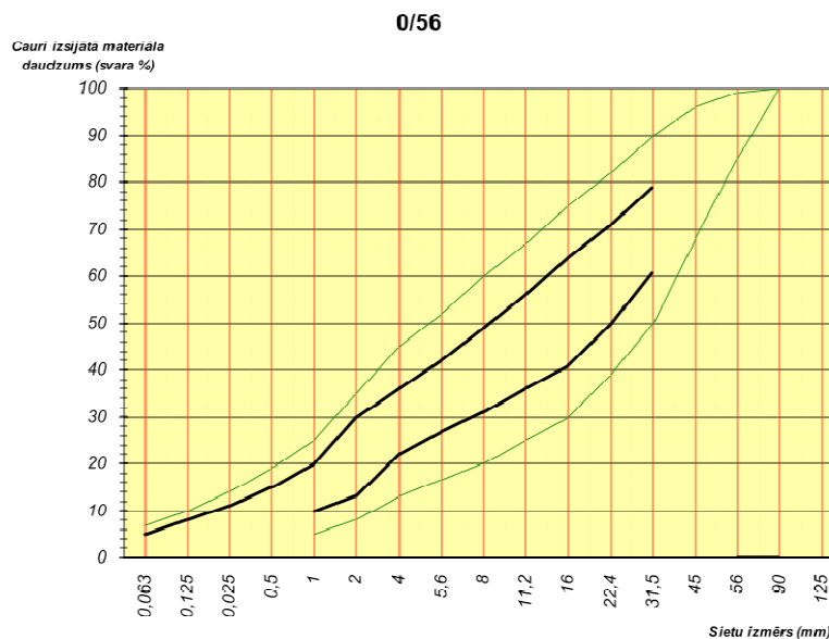
33. tabula. Prasības 0/56 maisījuma granulometriskajam sastāvam
