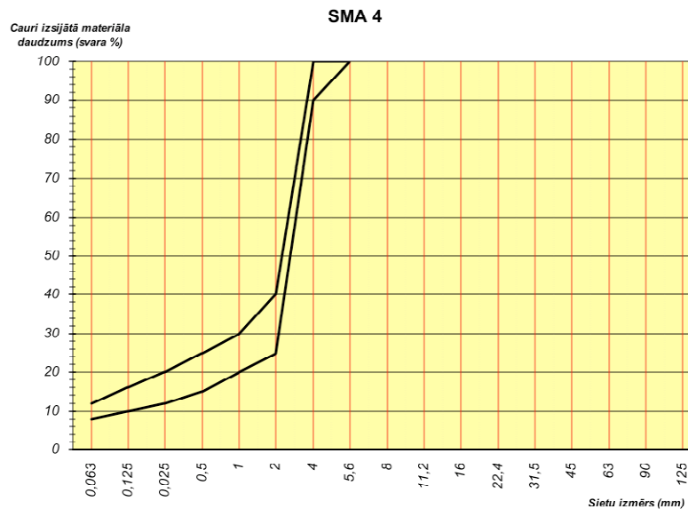
86. tabula. Prasības šķembu mastikas asfalta SMA 4 granulometriskajam sastāvam
