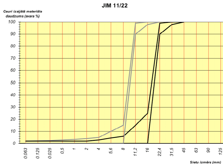
148. tabula. Prasības JIM 11/22 šķembu granulometriskajam sastāvam
