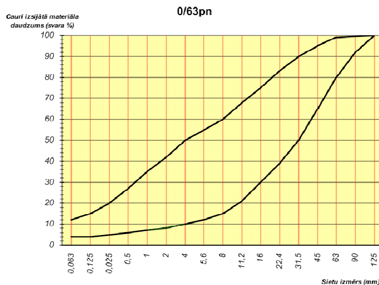
27. tabula. Prasības maisījuma 0/63pn granulometriskajam sastāvam
