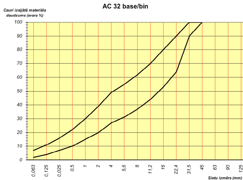
83. tabula. Prasības karstā asfalta AC 32 base/bin granulometriskajam sastāvam
