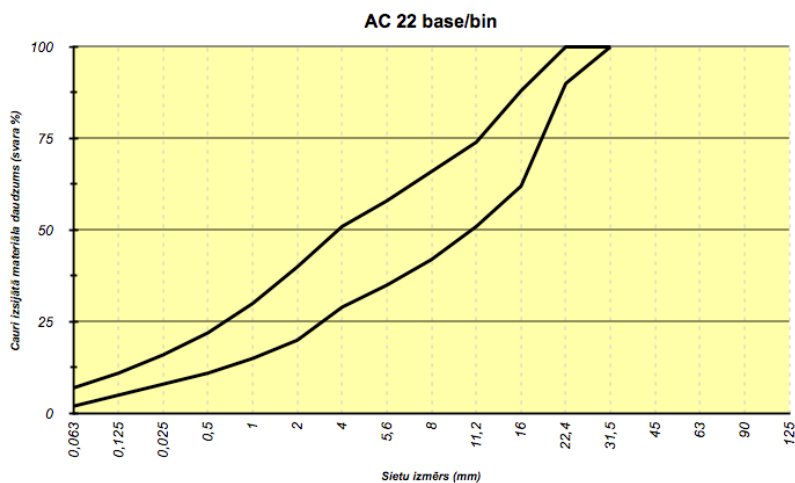
81. tabula. Prasības karstā asfalta AC 22 base/bin granulometriskajam sastāvam
