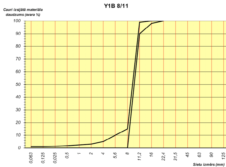
139. tabula. Prasības Y1B 8/11 granulometriskajam sastāvam
