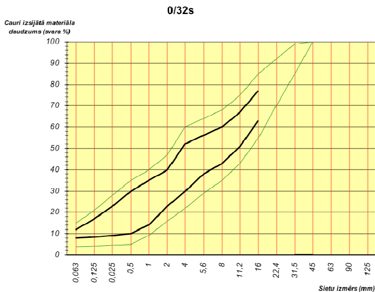
37. tabula. Prasības 0/32s maisījuma granulometriskajam sastāvam
