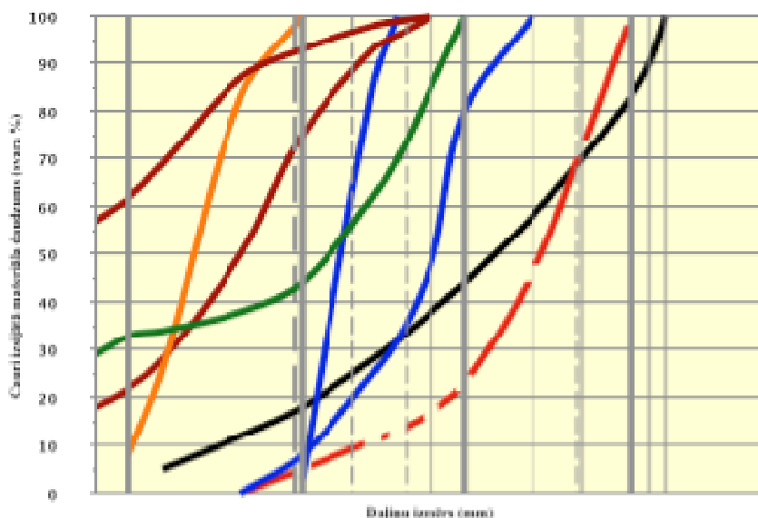
8. tabula. Grunšu granulometriskais sastāvs (informatīvi – grunšu raksturošanai)
