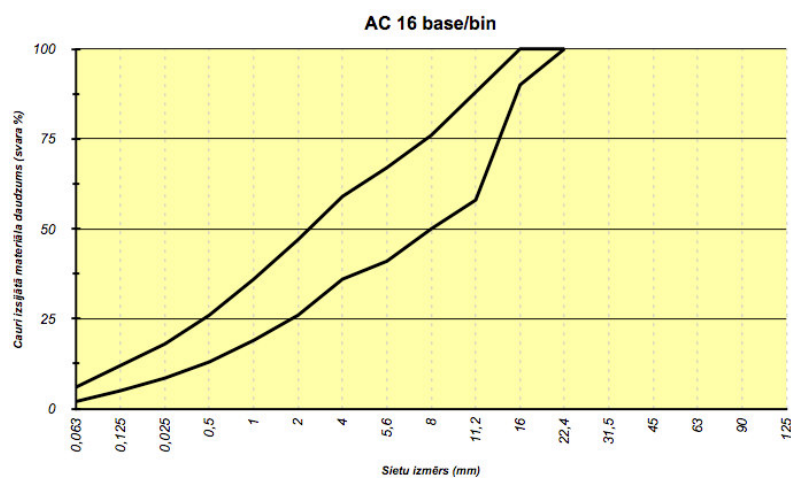
79. tabula. Prasības karstā asfalta AC 16 base/bin granulometriskajam sastāvam
