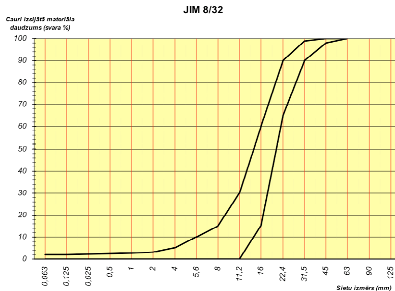
149. tabula. Prasības JIM 8/32 šķembu granulometriskajam sastāvam
