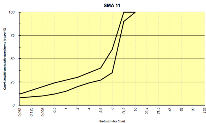
90. tabula. Prasības šķembu mastikas asfalta SMA 11 granulometriskajam sastāvam
