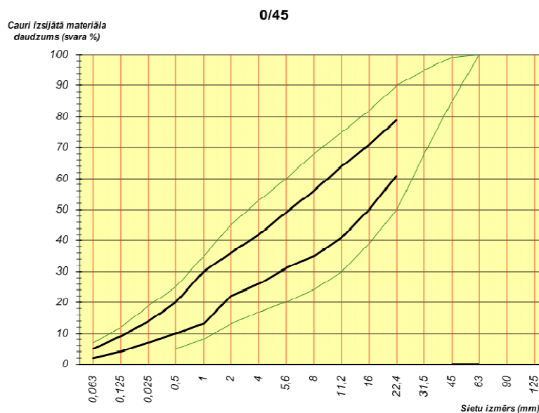
35. tabula. Prasības 0/45 maisījuma granulometriskajam sastāvam
