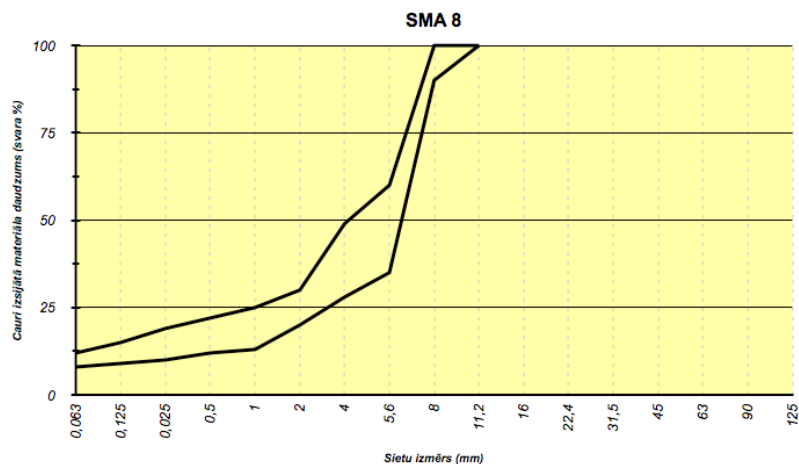
88. tabula. Prasības šķembu mastikas asfalta SMA 8 granulometriskajam sastāvam
