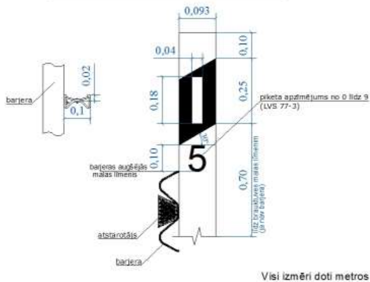
7.4-2 attēls. Signālstabiņi virs barjeras
