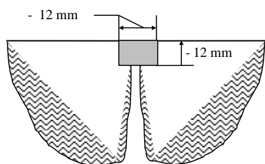
8.3-3 attēls. Ar hermētiķi aizpildīta plaisa
