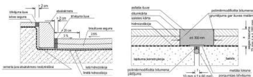
9.24-1 attēls. Blīvējuma šuve un mastikas (asfalta) šuve.
