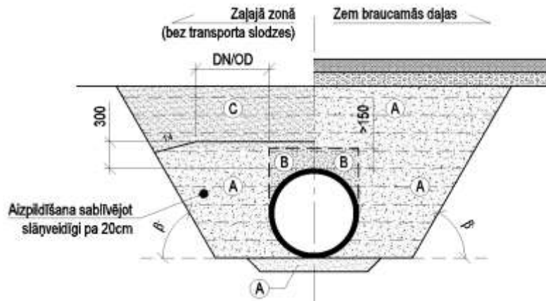
4.3-2 attēls. Caurtekas apbēruma sablīvējuma zonas.
