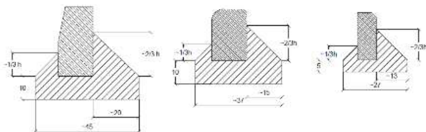
7.2-1 attēls. Betona apmaļu nostiprinājuma betonā skices
