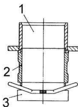
12.8-2 attēls. Triecienu blīvētāja tipiska blīvēšanas veidne
