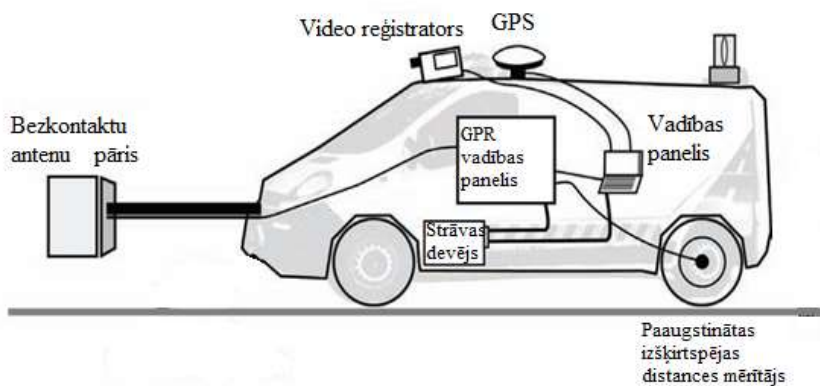
12.13-1 attēls. Mērījumiem izmantotā GPR iekārta
