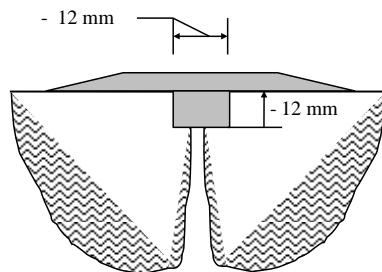
8.3-2 attēls. Ar hermētiķi aizlieta un aizpildīta plaisa
