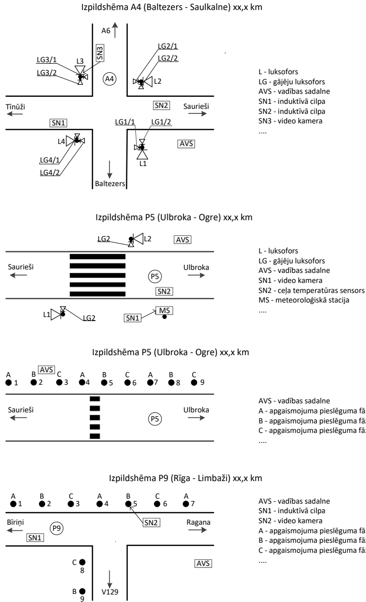
7.11-1 attēls. Izpildshēmas piemēri
