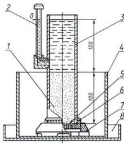
12.3-1 attēls. Smilšainu grunts filtrācijas koeficienta noteikšanas aparāts
