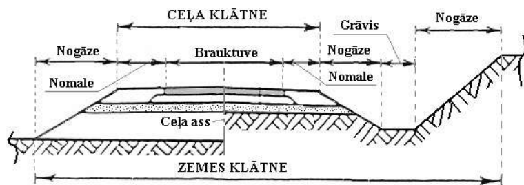
1.1-2 attēls. Ceļa konstrukcija
