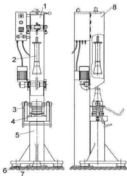
12.8-1 attēls. Triecienu blīvētāja shematisks attēls
