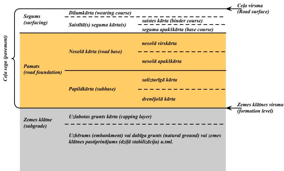
1.1-1 attēls. Ceļa konstruktīvās kārtas
