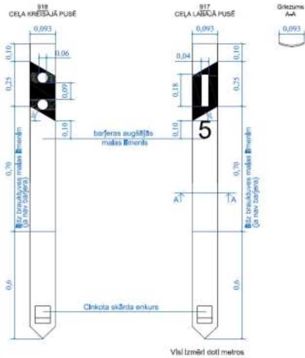
7.4-1 attēls. Signālstabiņi
