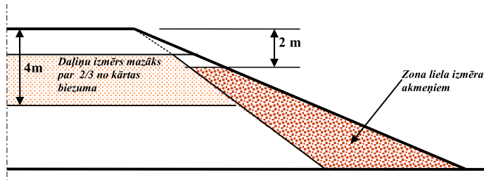
4.4-1 attēls. Zemes klātnes uzbēruma zonas
