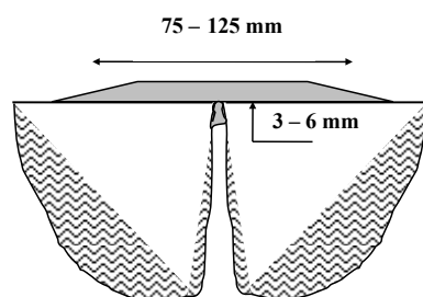
8.3-1 attēls. Ar hermētiķi aizlieta plaisa
