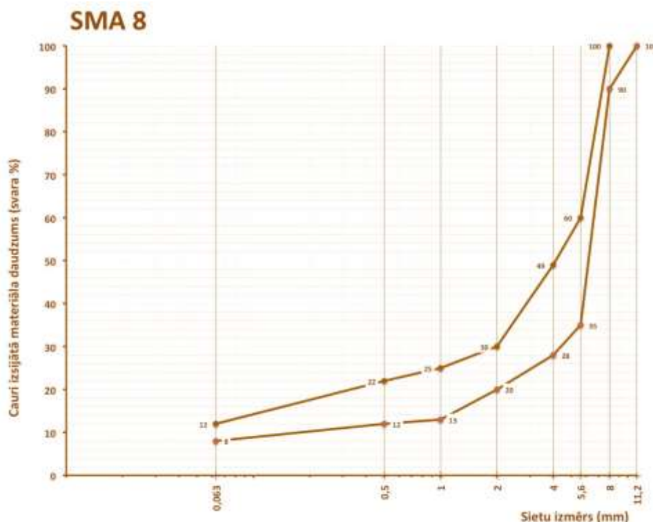
6.2-59 tabula. Prasības šķembu mastikas asfalta SMA 8 granulometriskajam sastāvam
