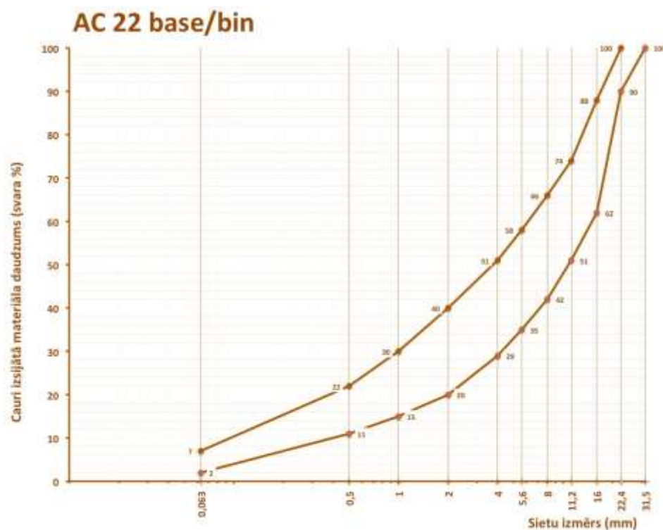
6.2-49 tabula. Prasības karstā asfalta AC 22 base/bin granulometriskajam sastāvam
