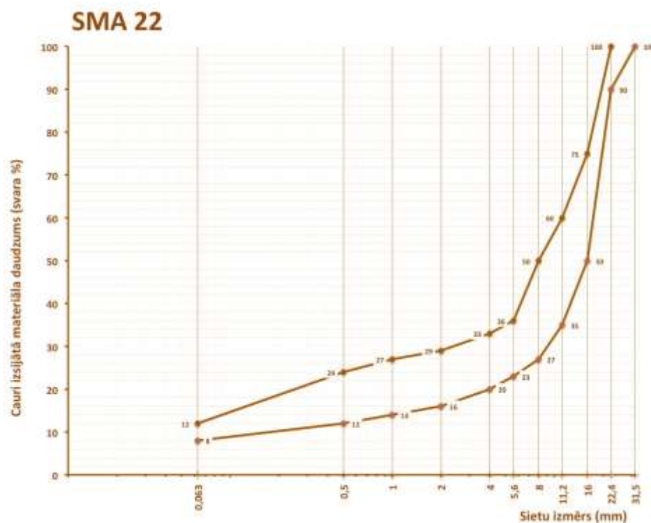
6.2-68 tabula. Prasības šķembu mastikas asfalta SMA 22 granulometriskajam sastāvam
