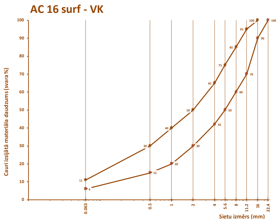
6.2-31 tabula. Prasības karstā asfalta AC 16 surf – VK granulometriskajam sastāvam
