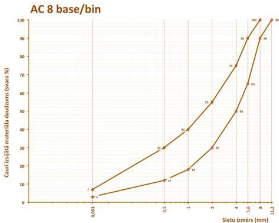
6.2-40 tabula. Prasības karstā asfalta AC 8 base/bin granulometriskajam sastāvam
