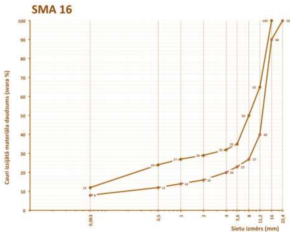
6.2-65 tabula. Prasības šķembu mastikas asfalta SMA 16 granulometriskajam sastāvam
