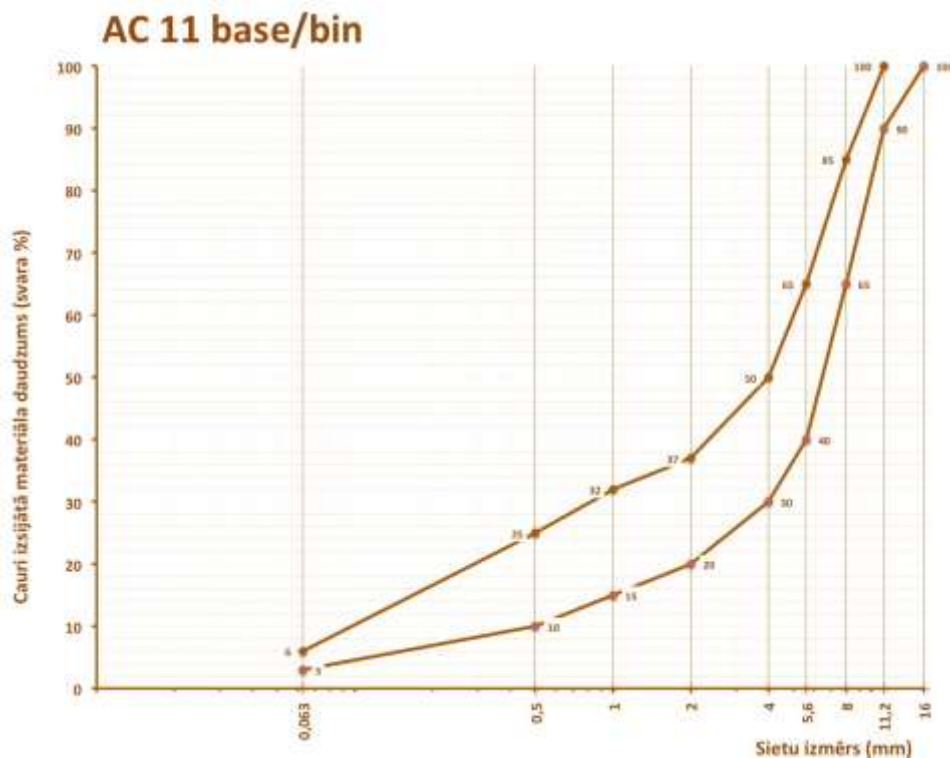
6.2-43 tabula. Prasības karstā asfalta AC 11 base/bin granulometriskajam sastāvam
