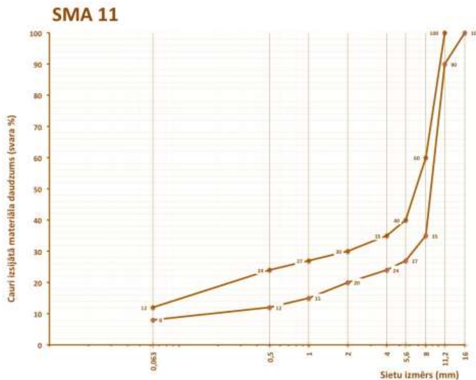
6.2-62 tabula. Prasības šķembu mastikas asfalta SMA 11 granulometriskajam sastāvam
