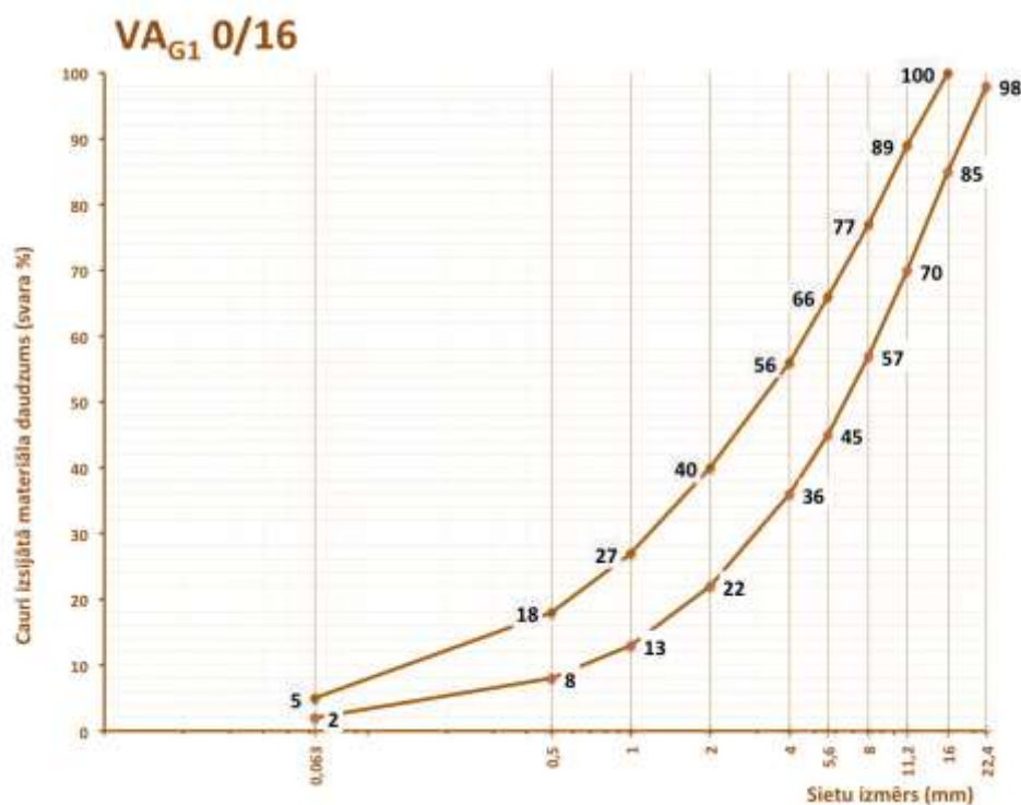
6.4-8 tabula. Prasības VA G1 0/16 granulometriskajam sastāvam
