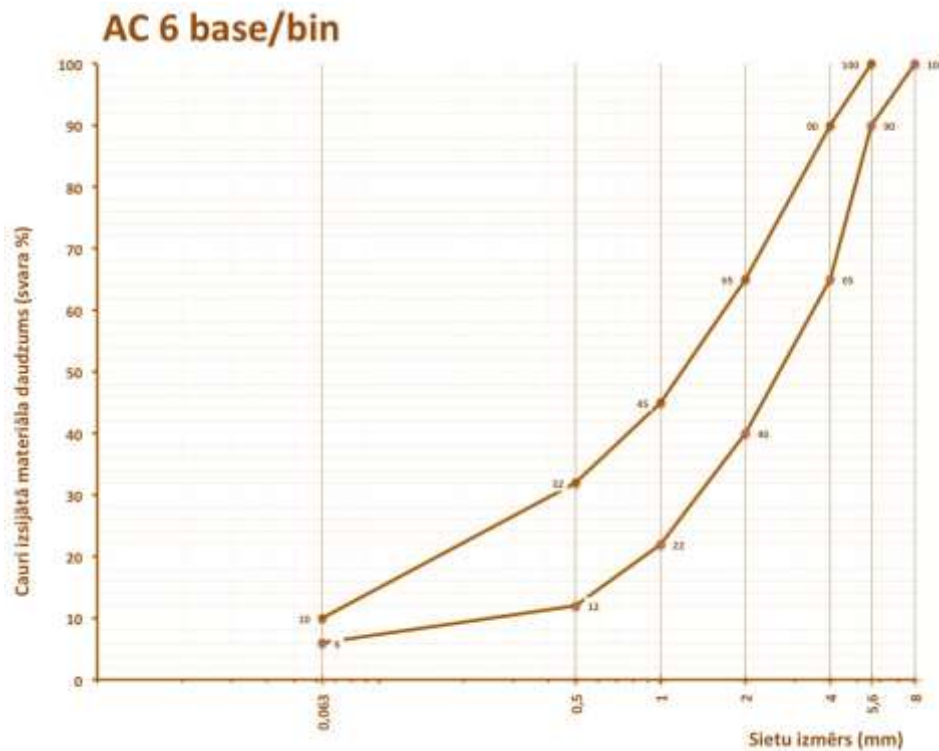
6.2-37 tabula. Prasības karstā asfalta AC 6 base/bin granulometriskajam sastāvam
