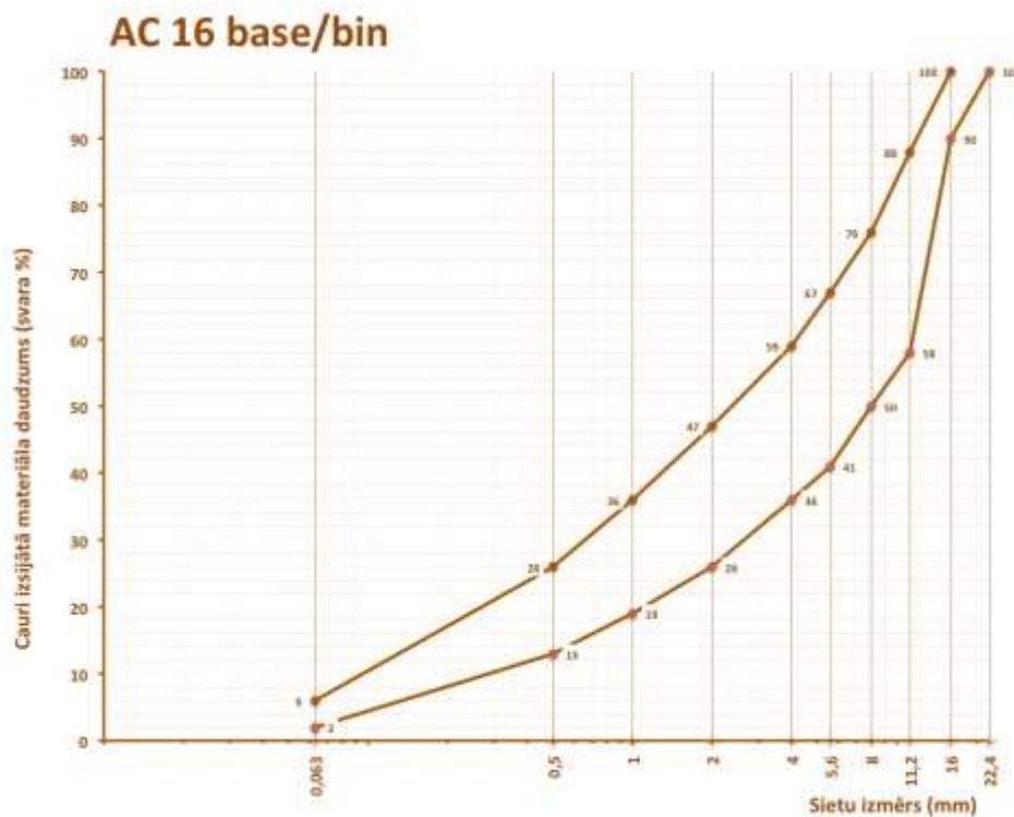
6.2-46 tabula. Prasības karstā asfalta AC 16 base/bin granulometriskajam sastāvam
