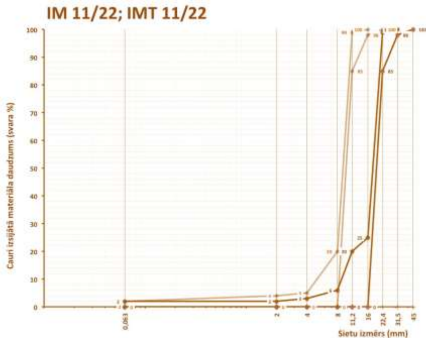
Šķembas 11/22 mm būvējamajai kārtai
